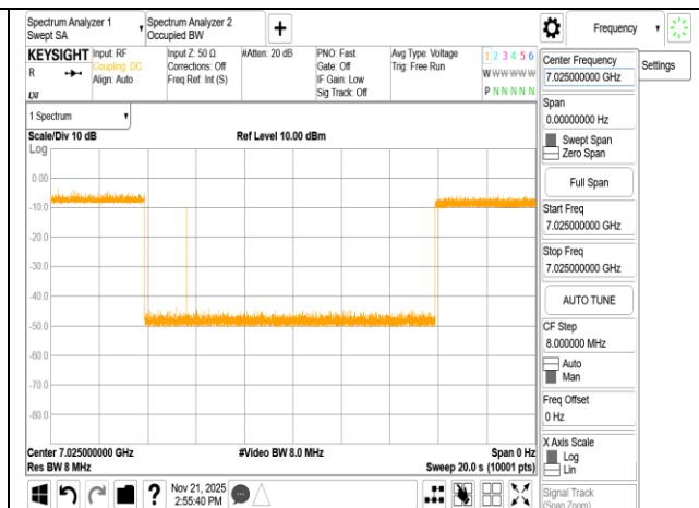
ax 80M 7025MHz Int7025MHz -72.6dBm Minimal
