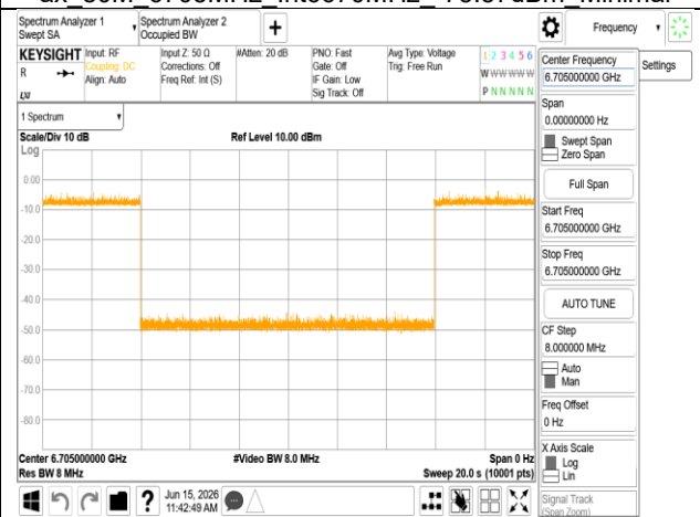
ax_80M_6705MHz_Int6705MHz_-76.05dBm OFF
