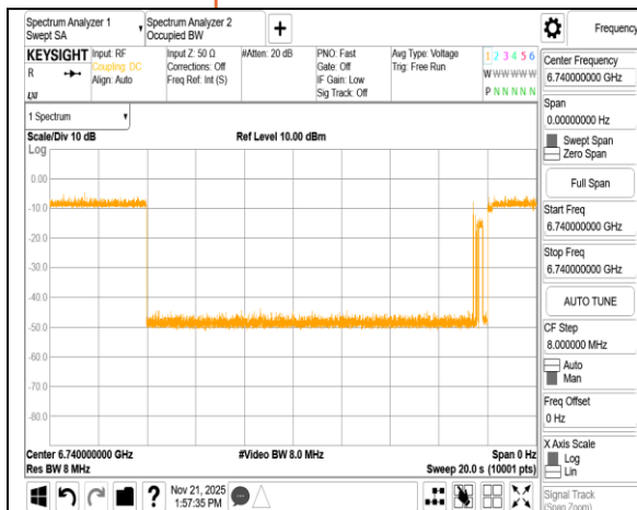
ax_80M_6705MHz_Int6740MHz_-75.72dBm OFF
