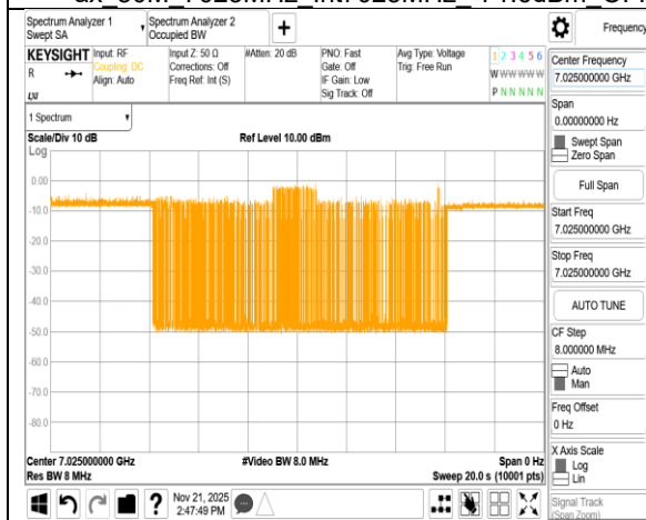
ax 80M 7025MHz Int7025MHz -78.6dBm ON
