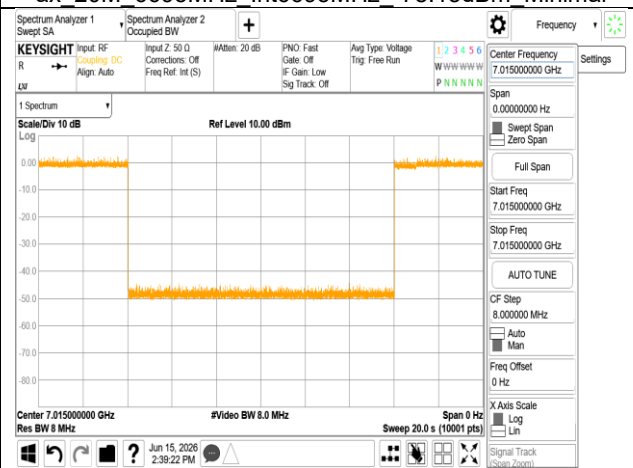
ax 20M 7015MHz Int7015MHz -76.13dBm OFF
