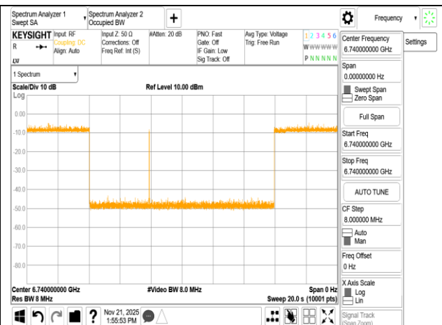
ax_80M_6705MHz_Int6740MHz_-76.72dBm Minimal
