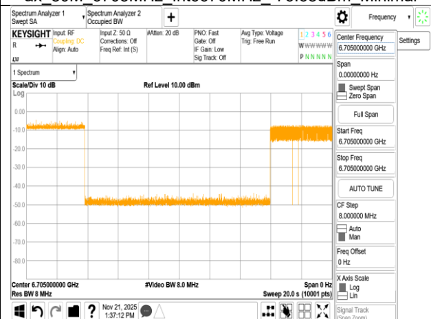
ax 80M_6705MHz_Int6705MHz_-69.75dBm OFF
