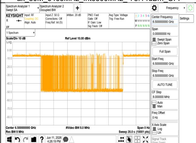
ax 80M_6465MHz_Int6500MHz_-77.14dBm_ON
