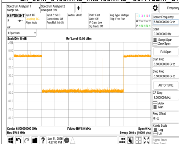
ax 80M_6465MHz_Int6500MHz_-76.14dBm_Minimal
