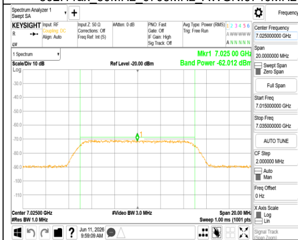
802.11ax 80MHz 7025MHz_AWGN:7025MHz
