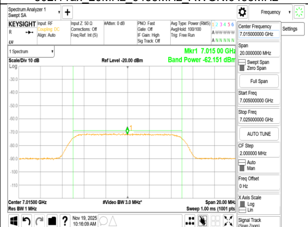
802.11ax 20MHz 7015MHz AWGN:7015MHz
