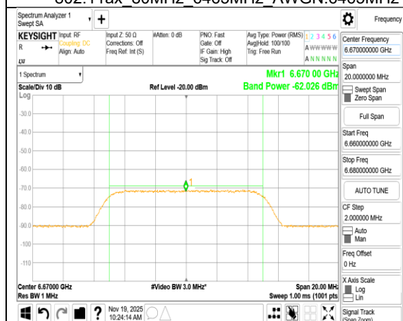
802.11ax 80MHz 6705MHz AWGN:6670MHz
