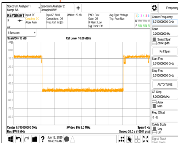
ax 80M_6705MHz_Int6740MHz_-75.19dBm OFF
