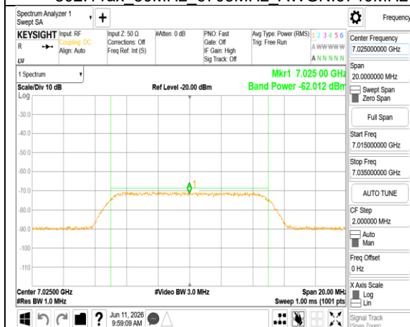
802.11ax 80MHz 7025MHz AWGN:7025MHz
