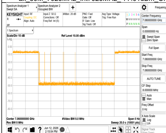
ax 80M 7025MHz Int7060MHz -75.14dBm Minimal
