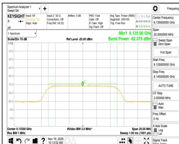
802.11ax 20MHz 6135MHz AWGN:6135MHz
