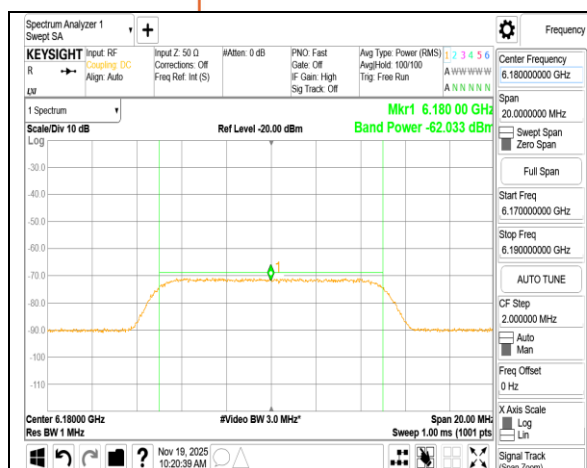
802.11ax 80MHz 6145MHz AWGN:6180MHz
