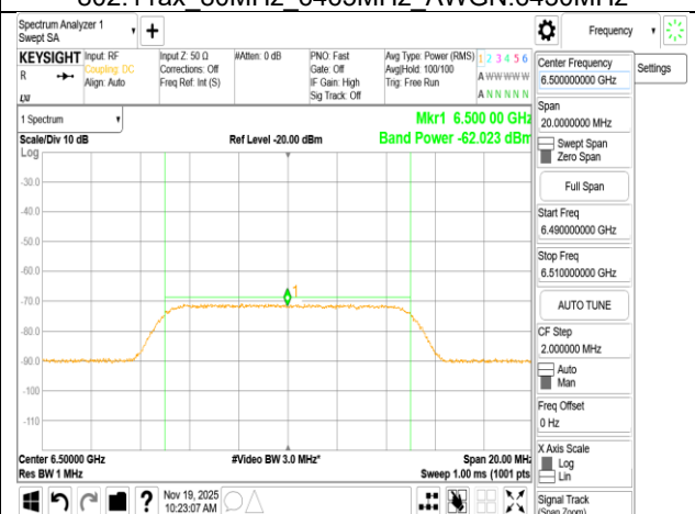
802.11ax 80MHz 6465MHz AWGN:6500MHz
