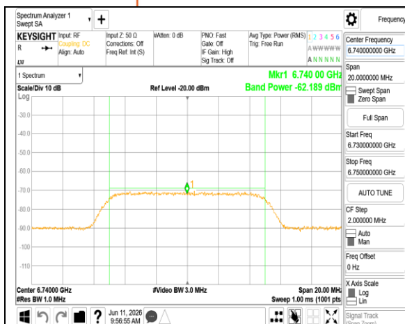
802.11ax 80MHz 6705MHz AWGN:6740MHz
