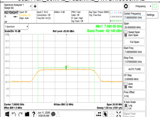
802.11ax 80MHz 7025MHz AWGN:7060MHz
