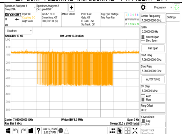
ax 80M 7025MHz Int7060MHz -76.14dBm ON
