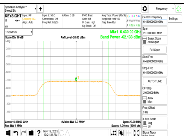
802.11ax 80MHz 6465MHz AWGN:6430MHz
