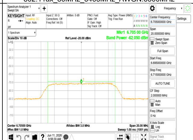
802.11ax 80MHz 6705MHz AWGN:6705MHz
