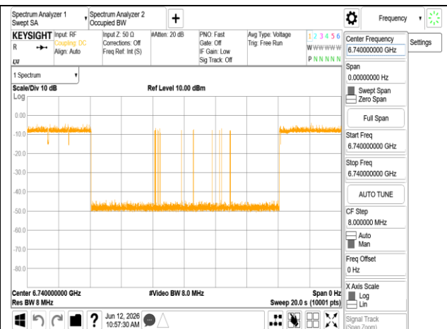
ax 80M_6705MHz_Int6740MHz_-76.19dBm Minimal
