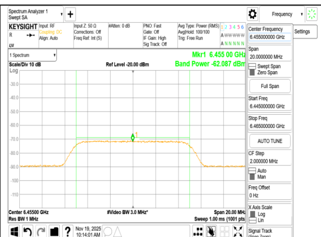
802.11ax 20MHz 6455MHz AWGN:6455MHz
