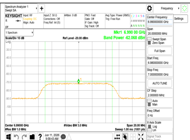
802.11ax 80MHz 7025MHz AWGN:6990MHz
