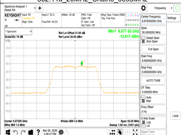
802.11a_20MHz_Chain0_6875MHz
