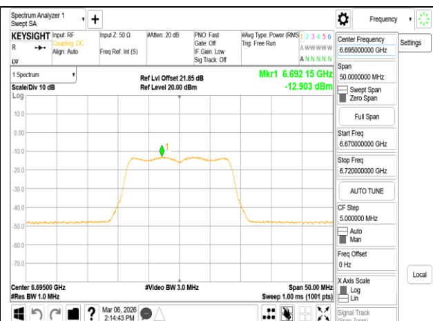
802.11a_20MHz_Chain0_6695MHz
