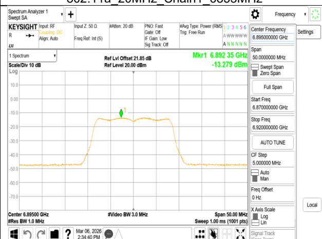
802.11a 20MHz Chain1 6895MHz
