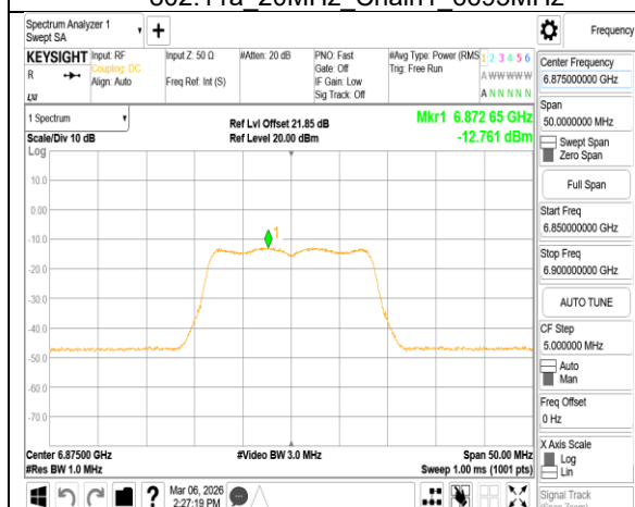
802.11a 20MHz Chain1 6875MHz
