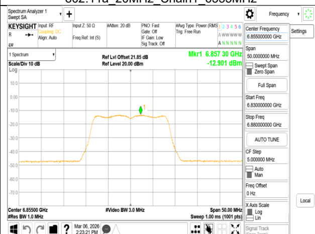
802.11a 20MHz Chain1 6855MHz
