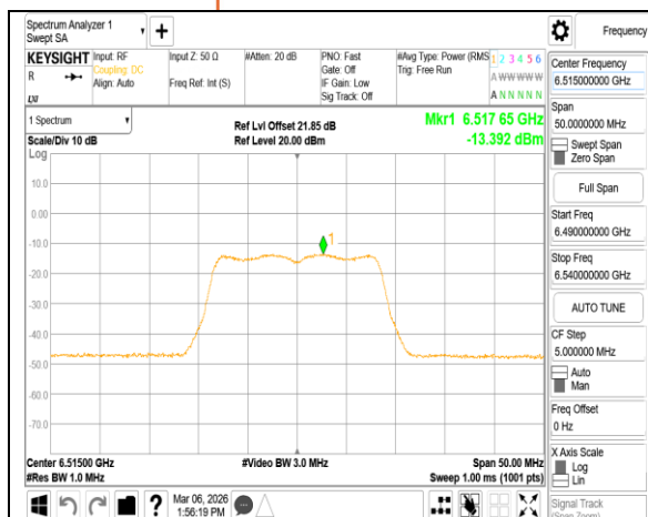
802.11a 20MHz Chain1 6515MHz
