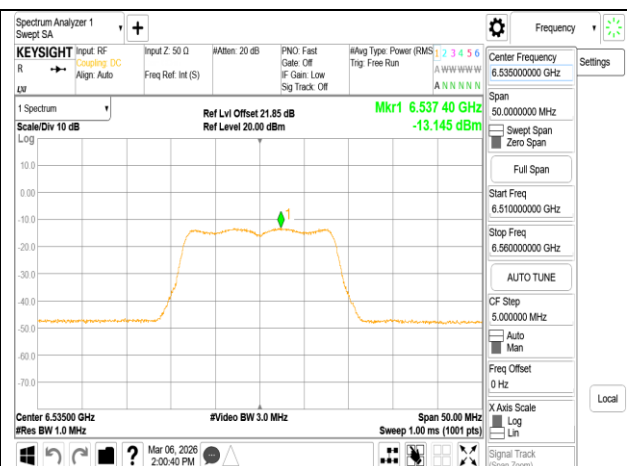
802.11a 20MHz Chain1 6535MHz
