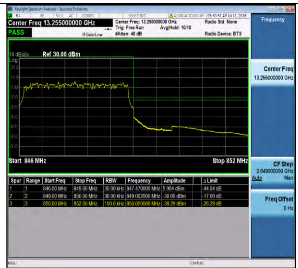
Band26(824-849)-3MHz-QPSK-27025-15RB#0-PASS
