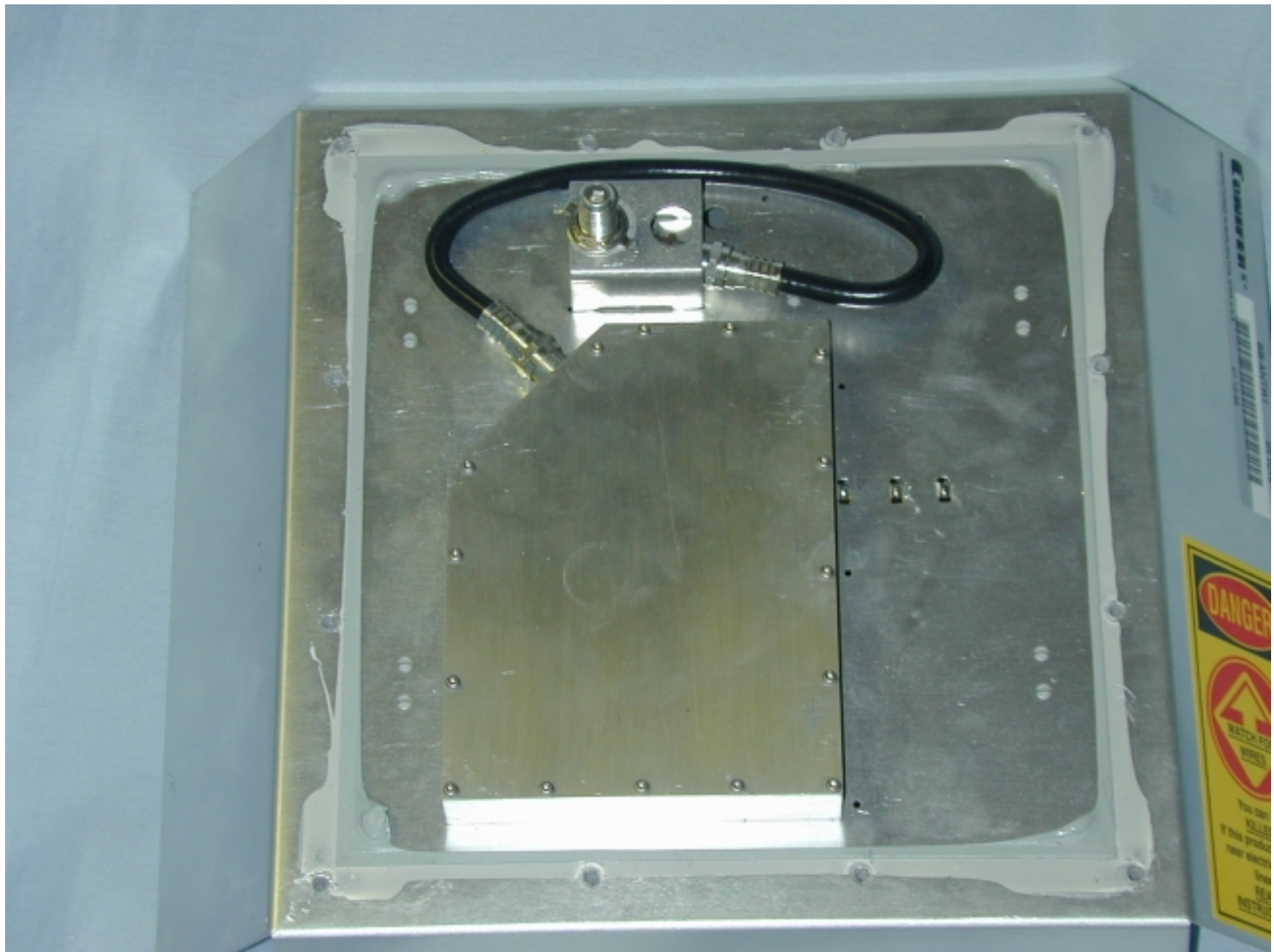
Photo 5 - Antenna Module
