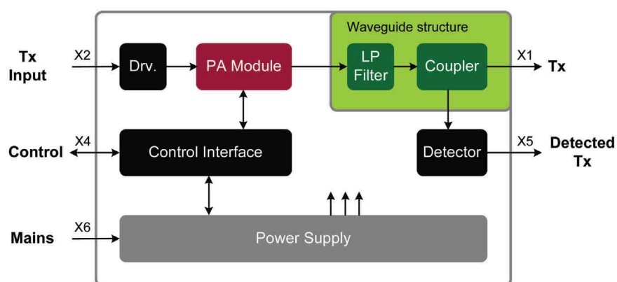
Fig. 4.7 SSPA 50 W
