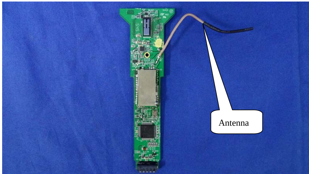
(4) EUT Photo
