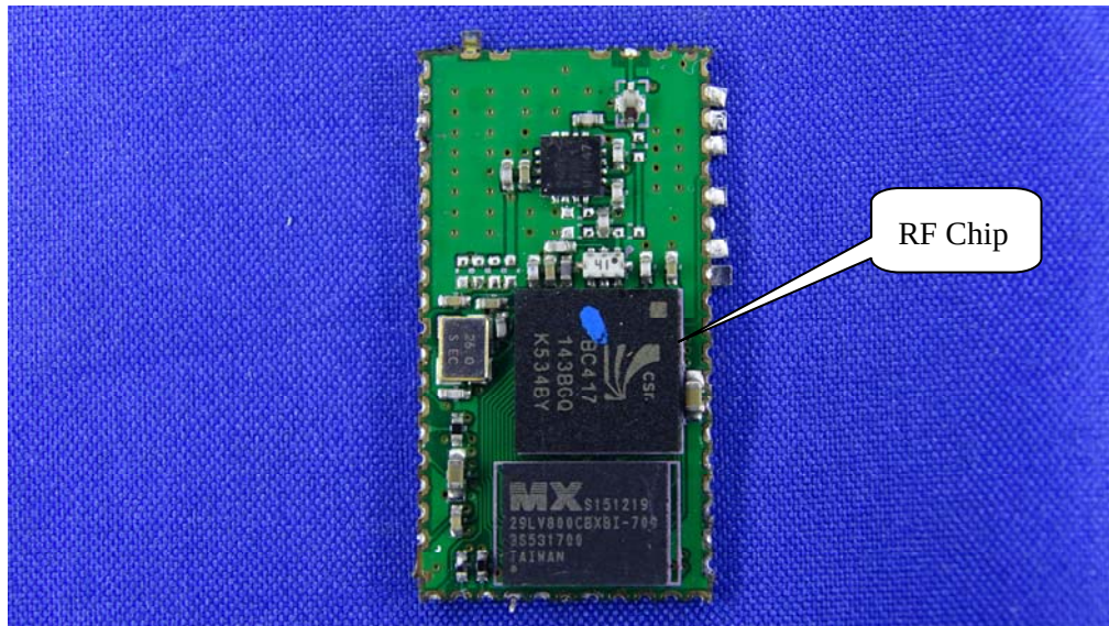
(8) EUT Photo
