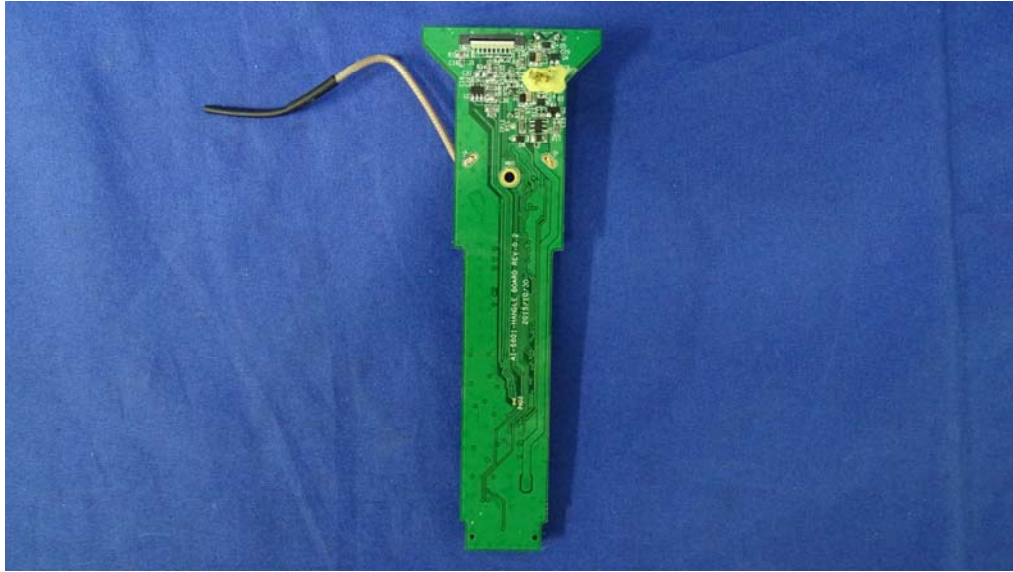
(5) EUT Photo
