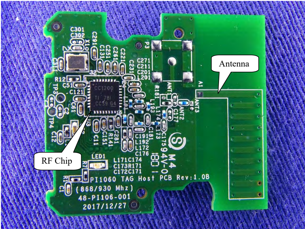
(20) EUT Photo (SUB 1G)
