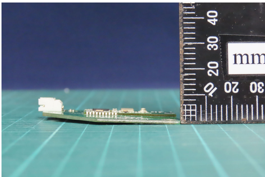
(6) EUT Photo
