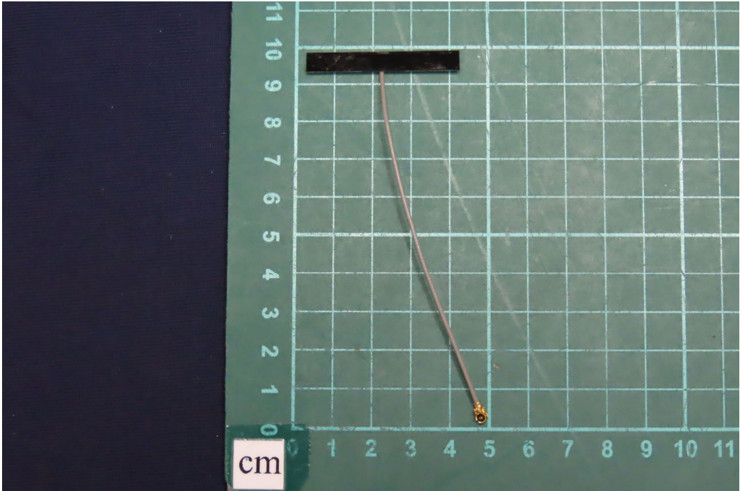
(8) EUT Photo_P/N: AA222 (PIFA Antenna)
