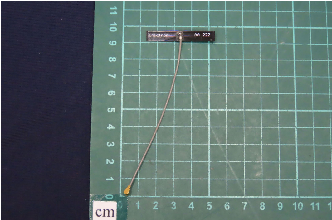
(7) EUT Photo_P/N: AA222 (PIFA Antenna)
