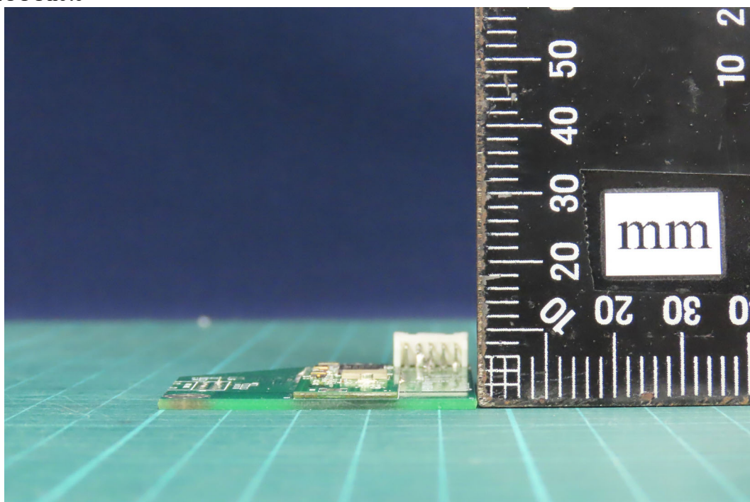
(3) EUT Photo
