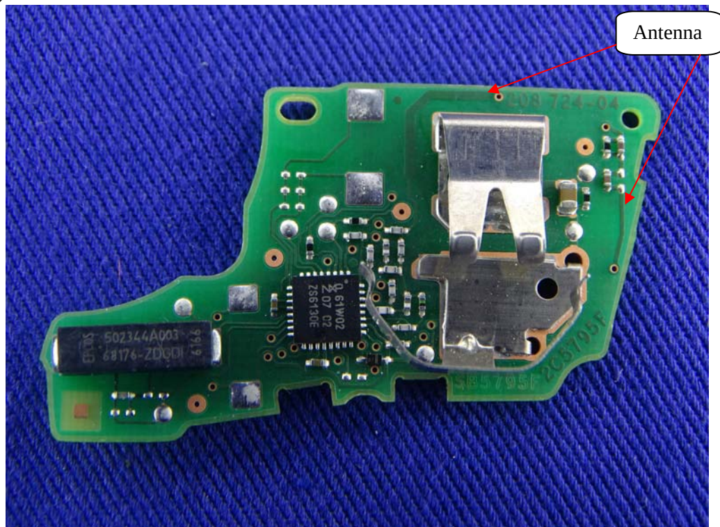
(16) EUT Photo
