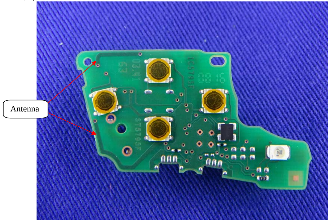
(17) EUT Photo
