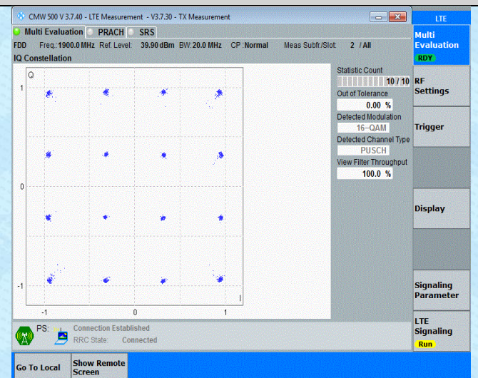
Band2-20MHz-16QAM-19100-27RB#0
