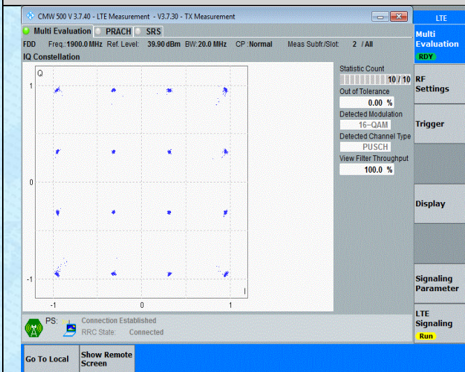
Band2-20MHz-16QAM-19100-27RB#73
