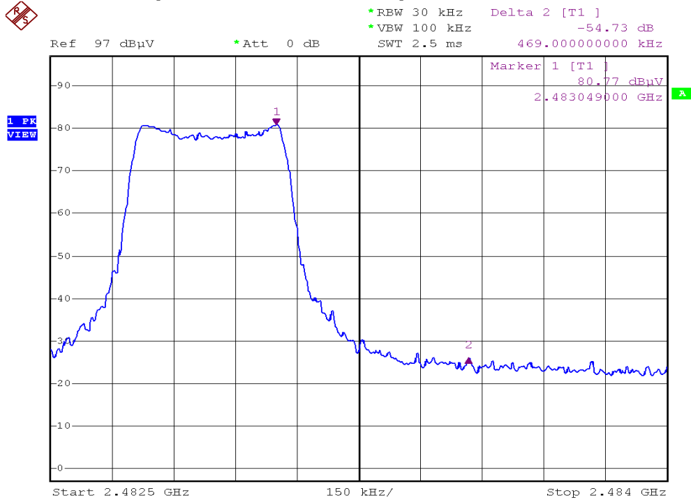
Plot B1B04 (KX-TG2132, 450mA)
