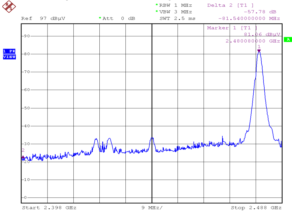
Plot B1A03 (KX-TG2132, 450mA)
