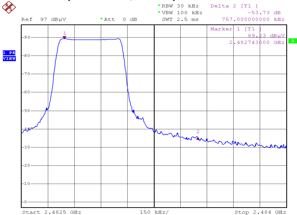
Plot B1B14 (KX-TG2132, 500mA)
