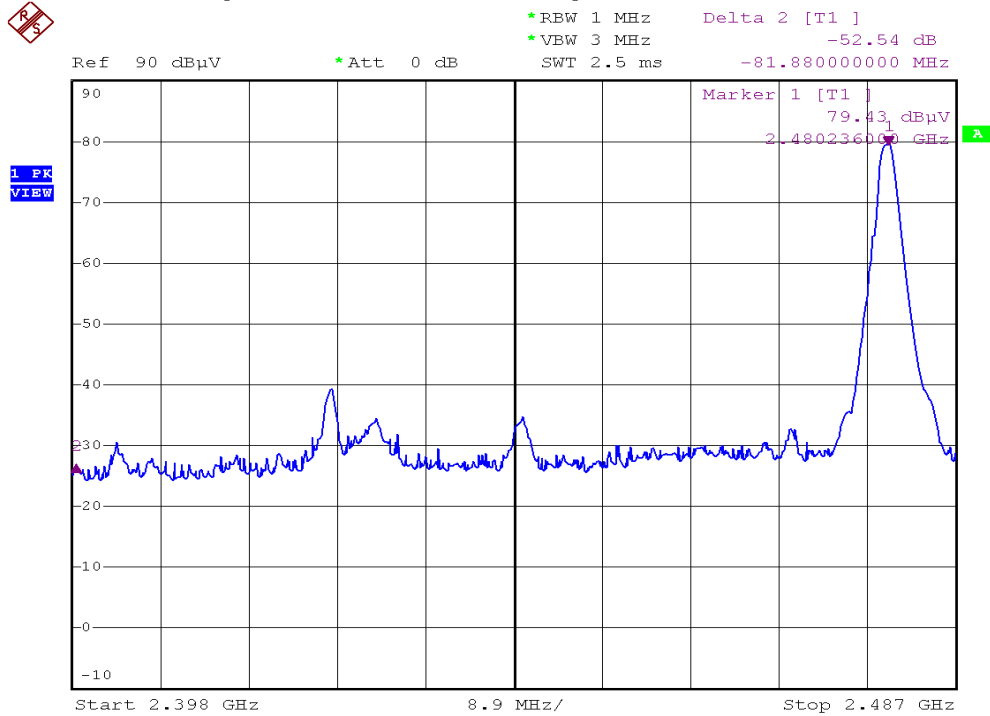
Plot B1A11 (KX-TG2130, 500mA)
