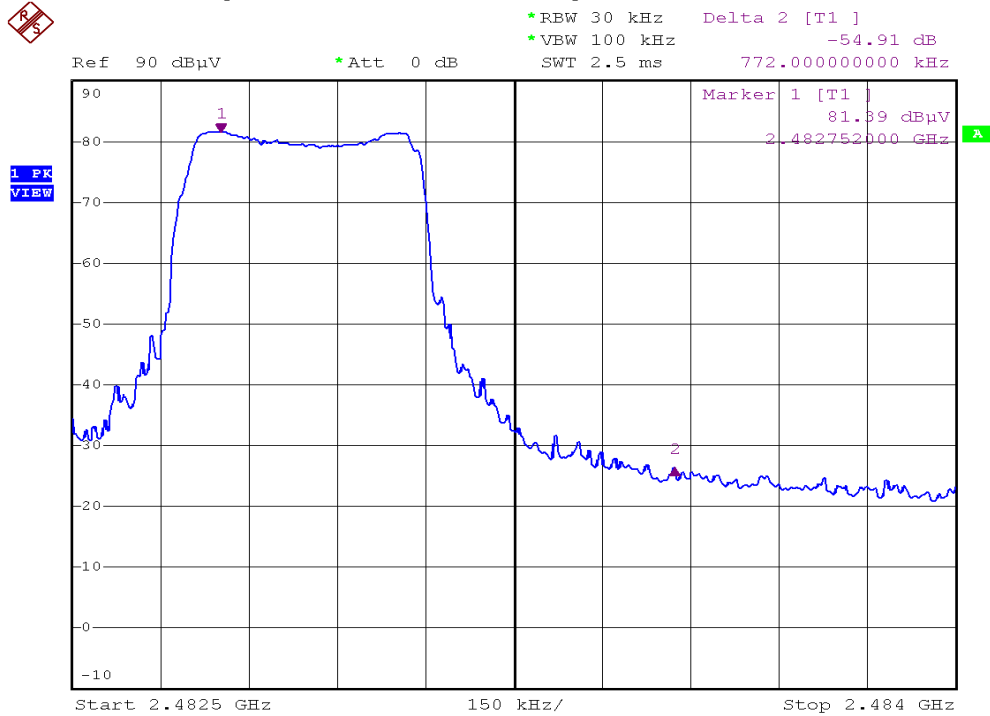
Plot B1B12 (KX-TG2130, 500mA)
