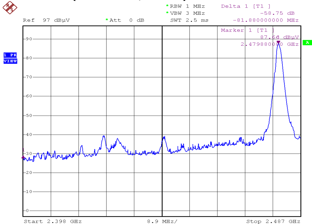
Plot B1A13 (KX-TG2132, 500mA)
