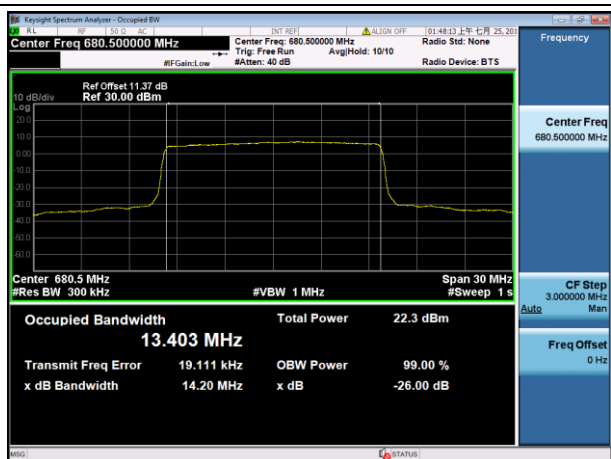
FDD71 MidRange 15 680.5 QPSK
