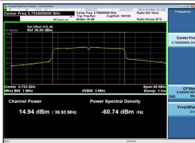
U-NII-3 Output Power-802.11n(40MHz) ,5755MHz,Ant1
