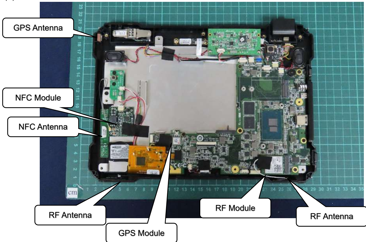
(8) EUT Photo
