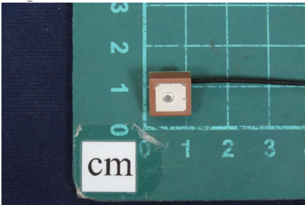
(25) EUT Photo_GPS Antenna
