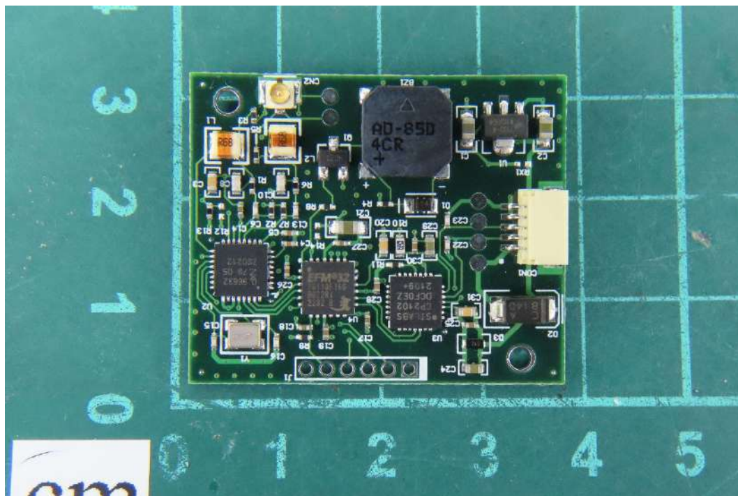
(12) EUT Photo
