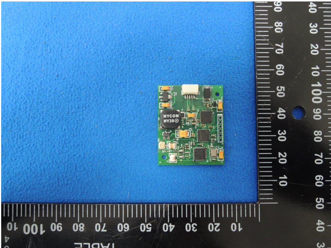
RFID Module
