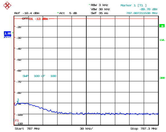
776-787MHz 2 x MSK ≤ AGC Upper
