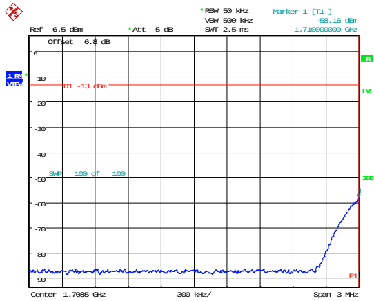
1710-1755MHz 1 x AWGN AGC +3dB lower
