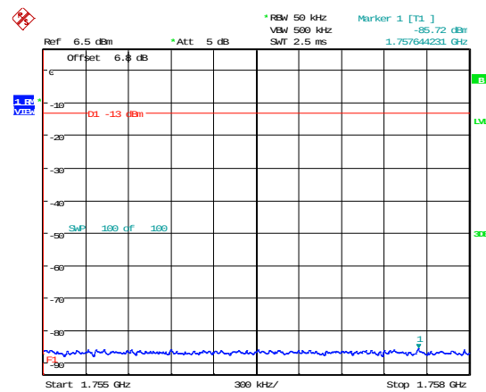
1710-1755MHz 2 x AWGN \leq AGC Upper
