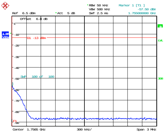
1710-1755MHz 1 x AWGN \leq AGC Upper
