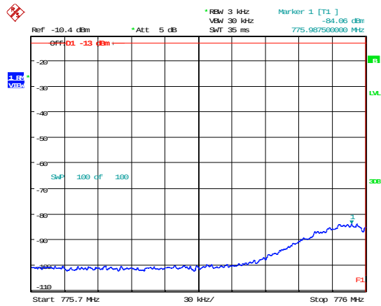
776-787MHz 2 x MSK AGC +3dB lower
