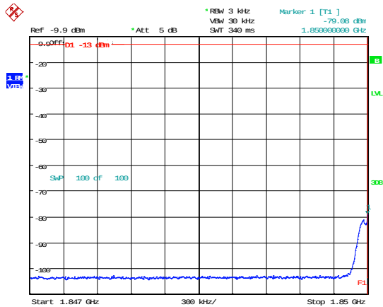
1850-1915MHz 1 x MSK AGC +3dB lower
