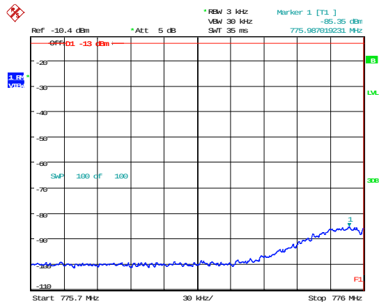
776-787MHz 2 x MSK ≤ AGC lower
