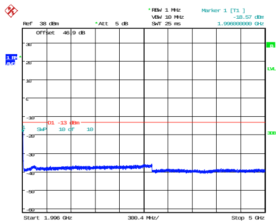
1930-1995MHz Mid AWGN 1.996-5GHz
