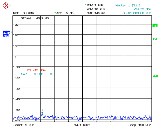
1930-1995MHz Mid AWGN 9-150 kHz
