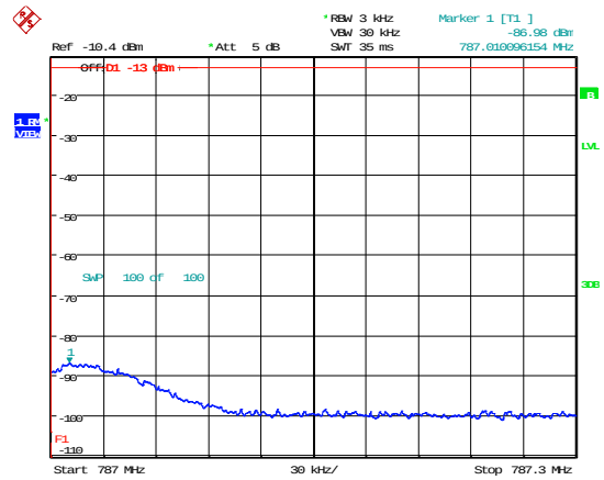
776-787MHz 2 x MSK AGC +3dB upper
