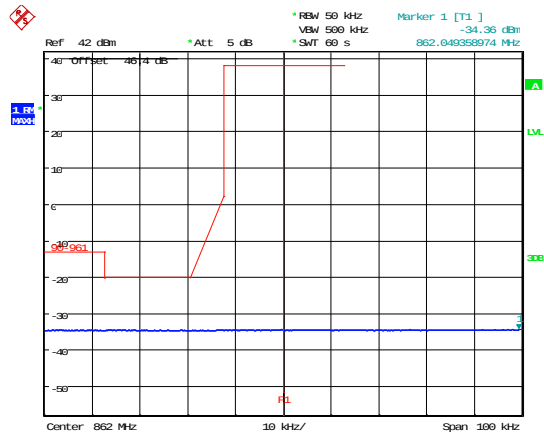
Bottom WCDMA AGC
