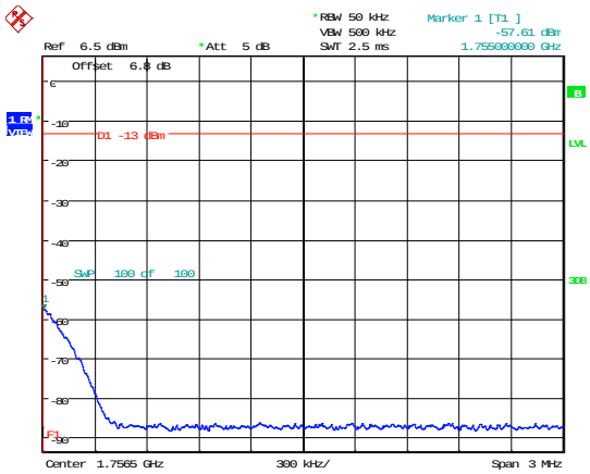
1710-1755MHz 1 x AWGN AGC +3dB upper
