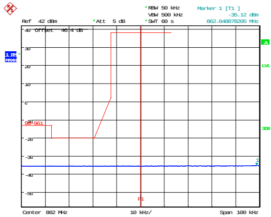
Bottom WCDMA AGC+3
