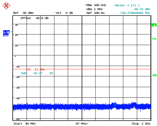
1930-1995MHz Mid AWGN 30-1MHz
