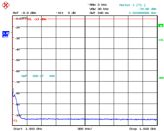
1850-1915MHz 1 x MSK AGC +3dB upper
