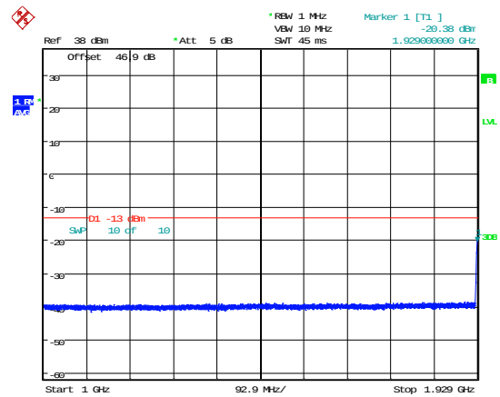
1930-1995MHz Mid AWGN 1-1.929GHz
