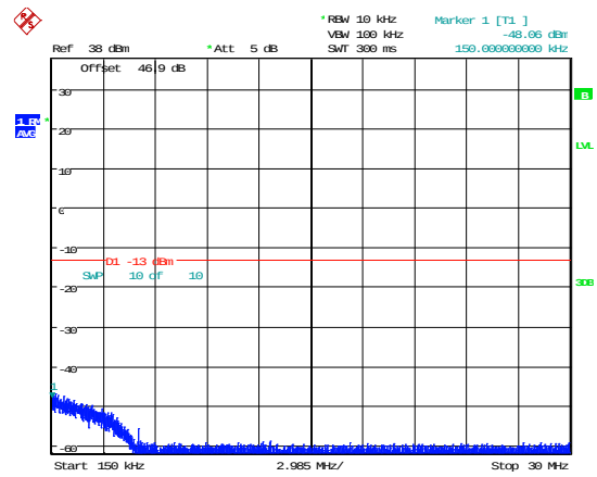
1930-1995MHz Mid AWGN 150 kHz-30MHz
