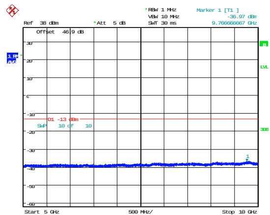
1930-1995MHz Mid AWGN 5-10GHz
