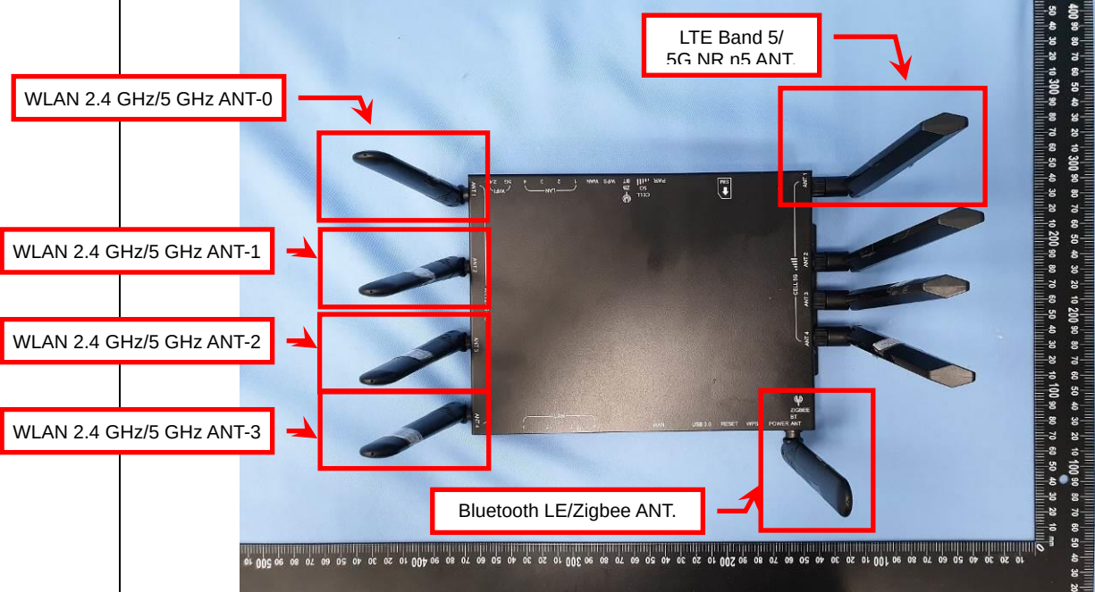
EUT Photo (2)
