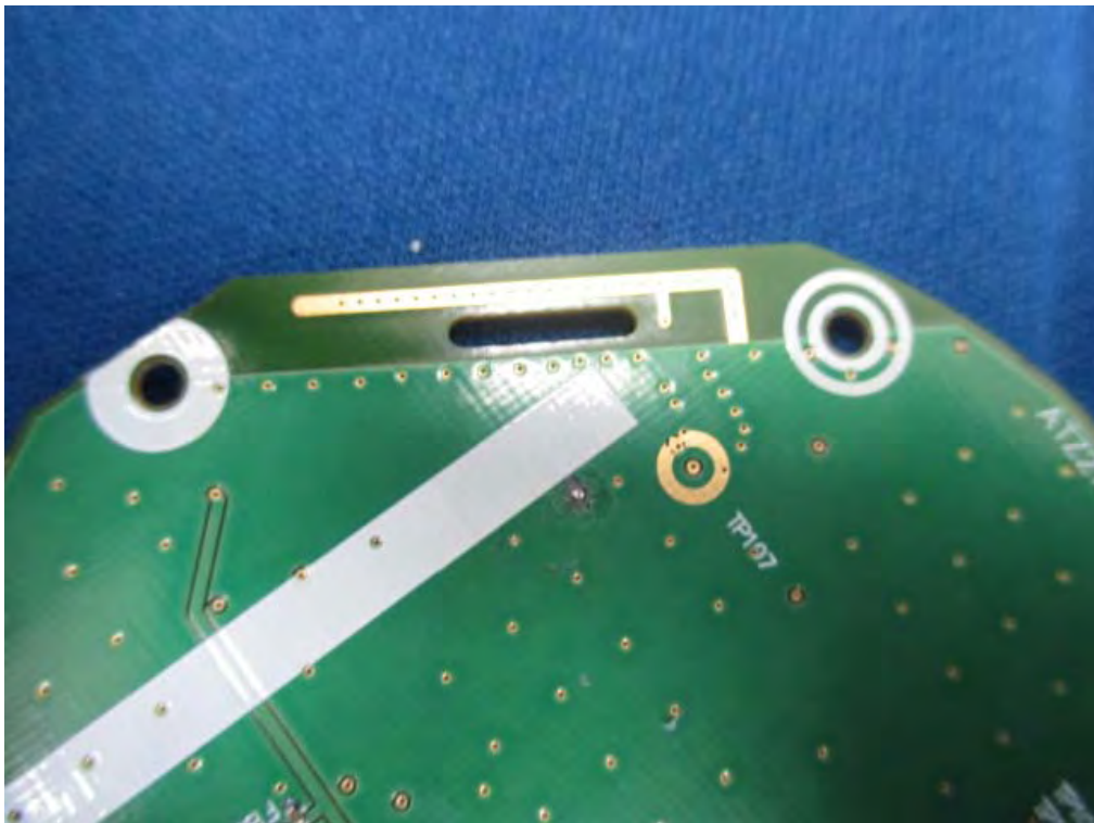
(20) EUT Photo (Antenna)
