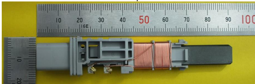
Bottom
