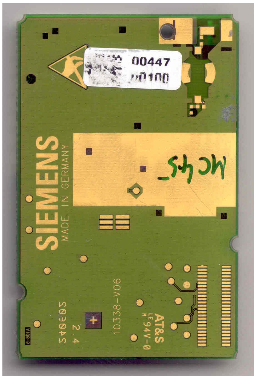
GSM Module Bottom view
