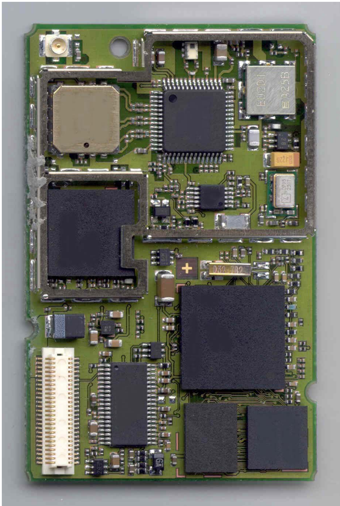
GSM Module Top view
