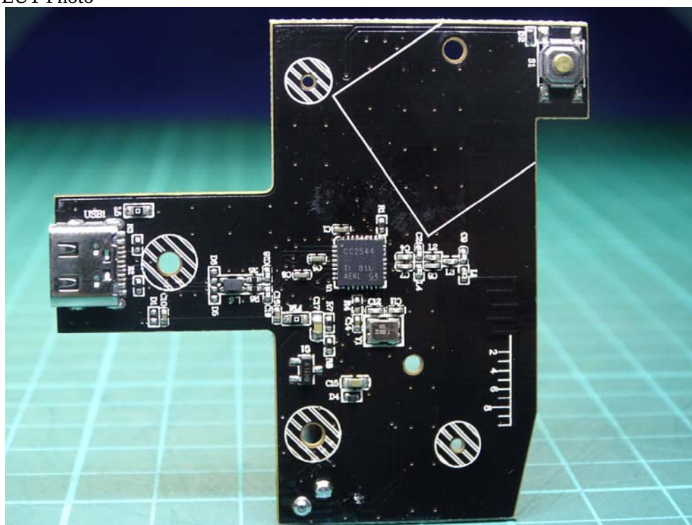
(18) EUT Photo
