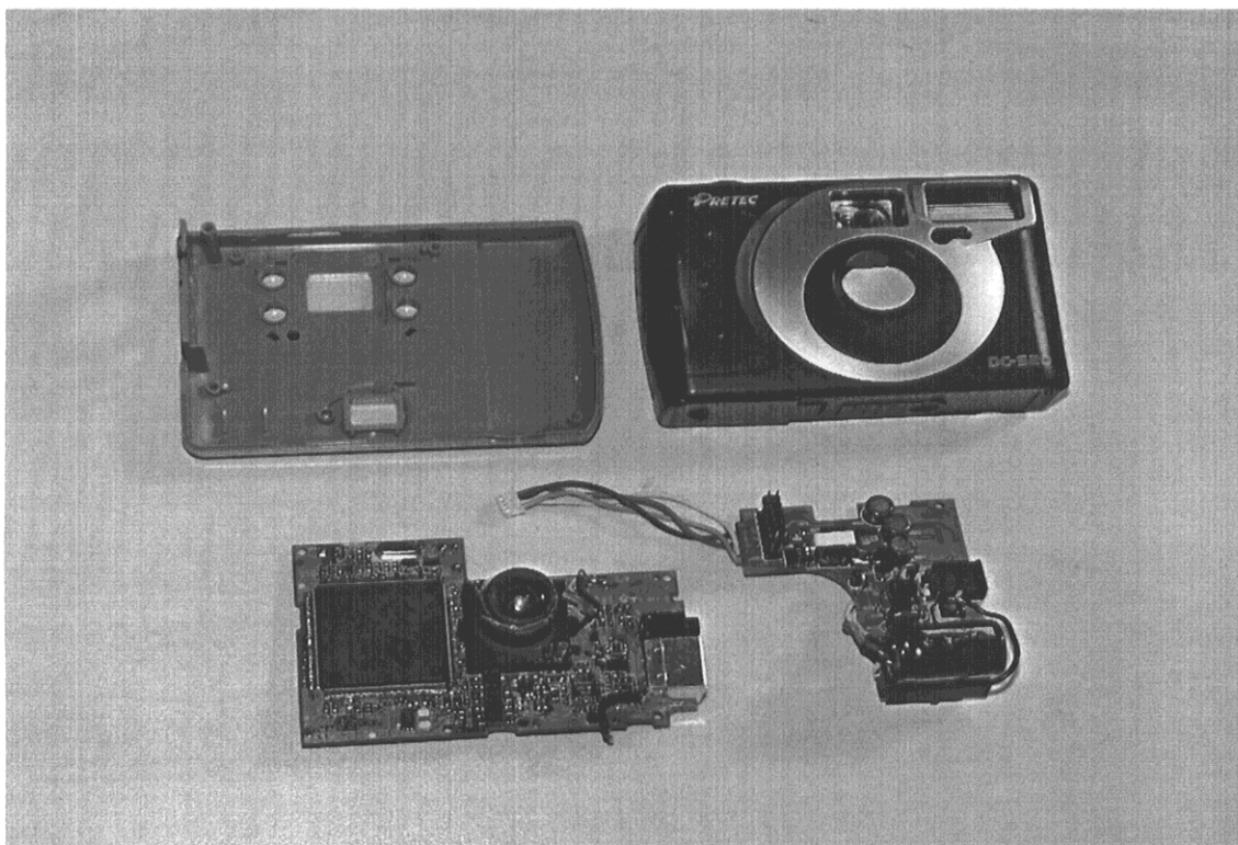
(6) EUT Photo
