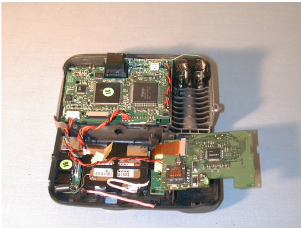
(24) EUT Photo
