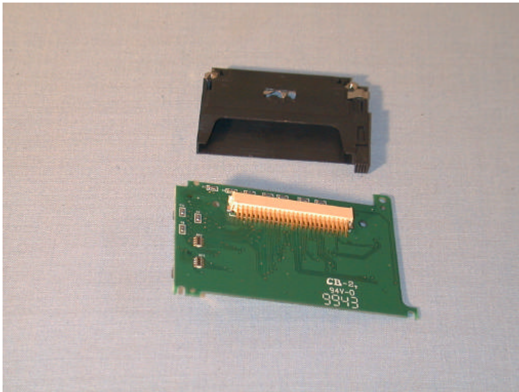
(48) EUT Photo
