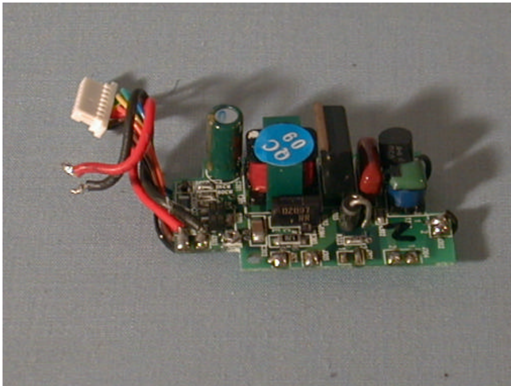
(50) EUT Photo
