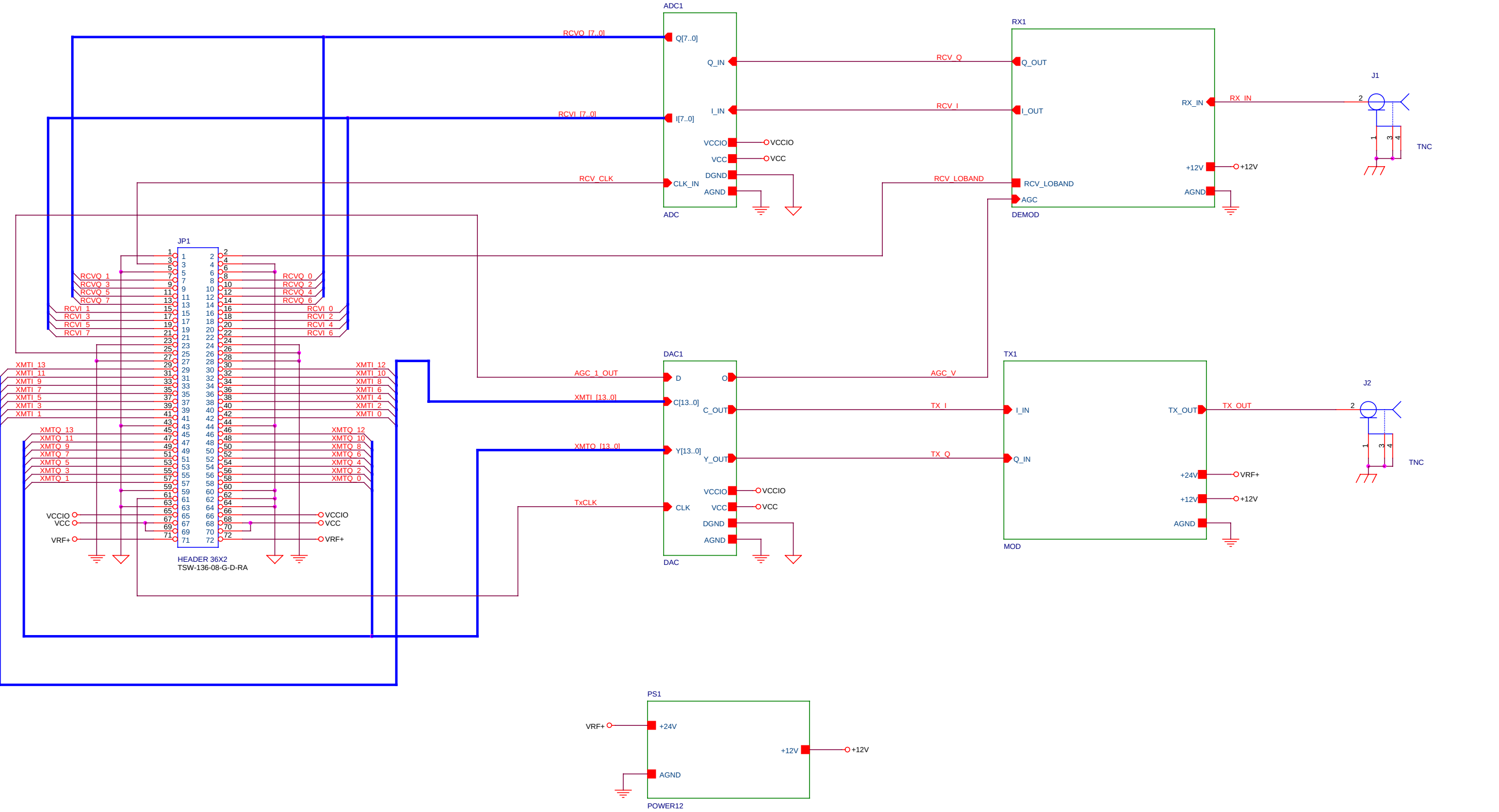
Z_PCB1 IO4_IF PCB
