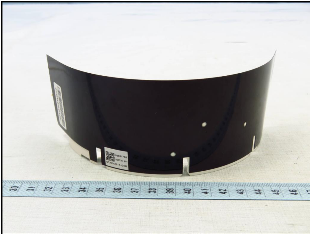
Antenna: A21LG2-R
