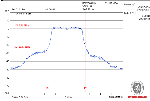
802.11a_CH48
