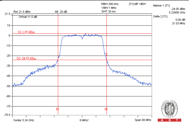
802.11n (HT20)_CH48
