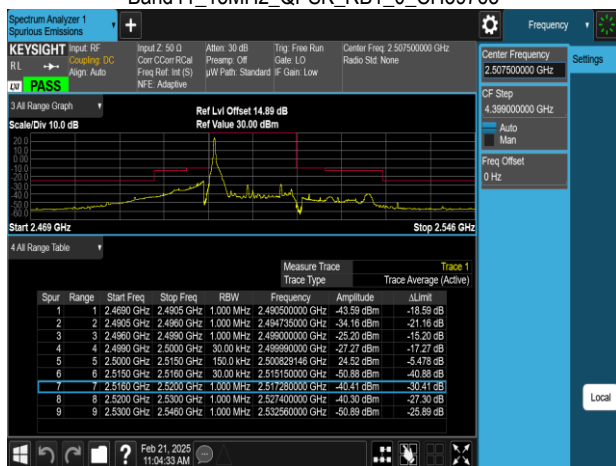
Band41_15MHz_QPSK_RB1_74_CH39765
