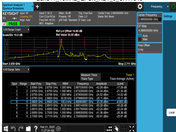
Band41_10MHz_QPSK_RB1_49_CH41540
