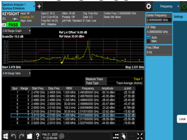
Band41_10MHz_QPSK_RB1_49_CH39740
