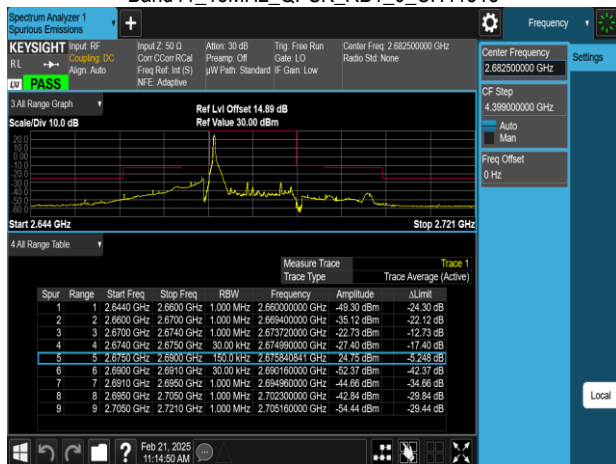
Band41_15MHz_QPSK_RB1_74_CH41515
