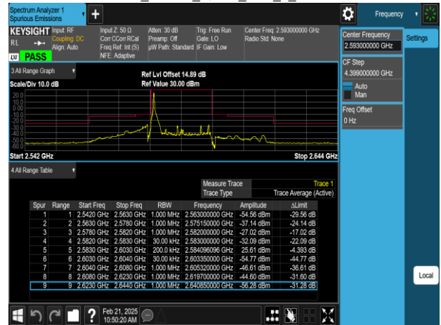
Band41_20MHz_QPSK_RB1_99_CH40620
