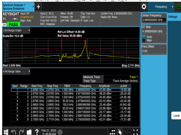
Band41_10MHz_QPSK_RB1_49_CH41540
