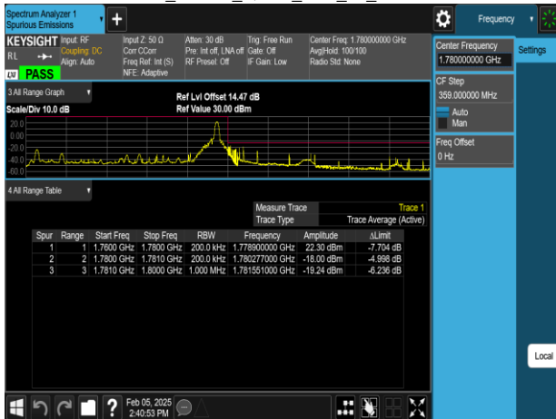
Band66 20MHz_QPSK_RB1_99_CH132572
