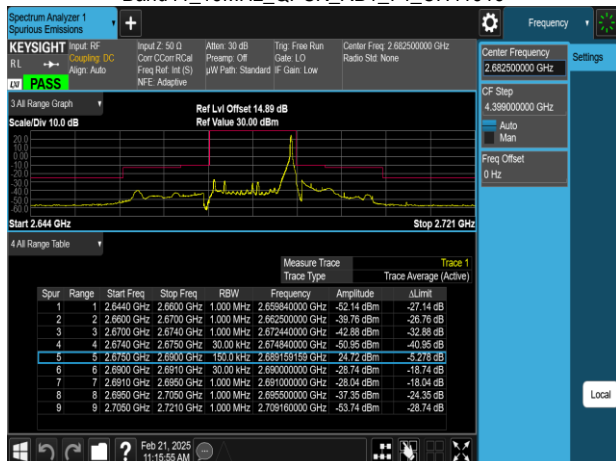
Band41_15MHz_QPSK_RB1_74_CH41515
