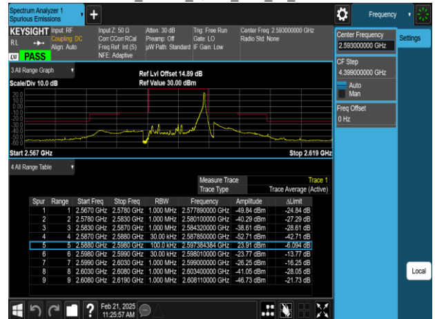
Band41_10MHz_QPSK_RB1_49_CH40620
