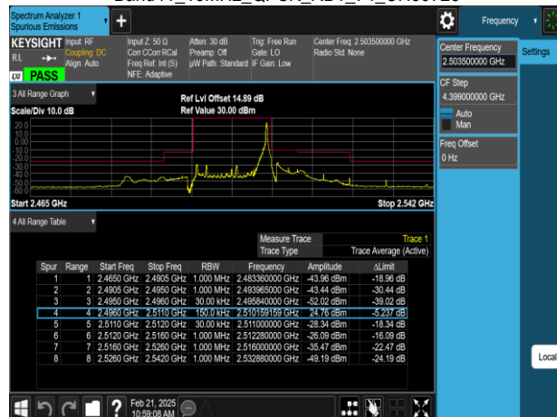
Band41_15MHz_QPSK_RB1_74_CH39725
