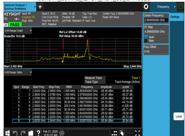
Band41_20MHz_QPSK_RB1_99_CH40620
