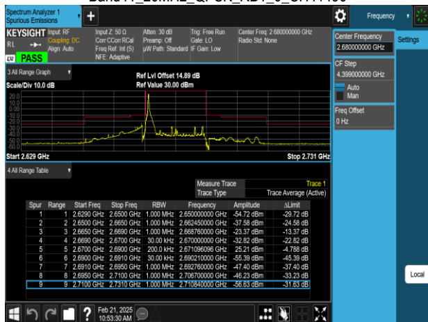
Band41 20MHz QPSK RB1_99 CH41490
