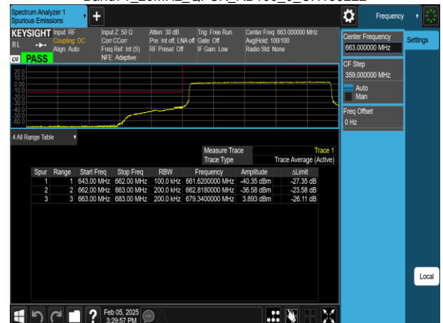
Band71_20MHz_QPSK_RB100_0_CH133222
