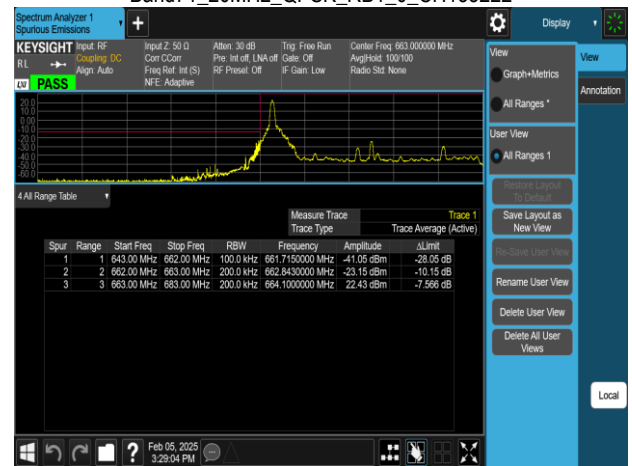
Band71_20MHz_QPSK_RB100_0_CH133222
