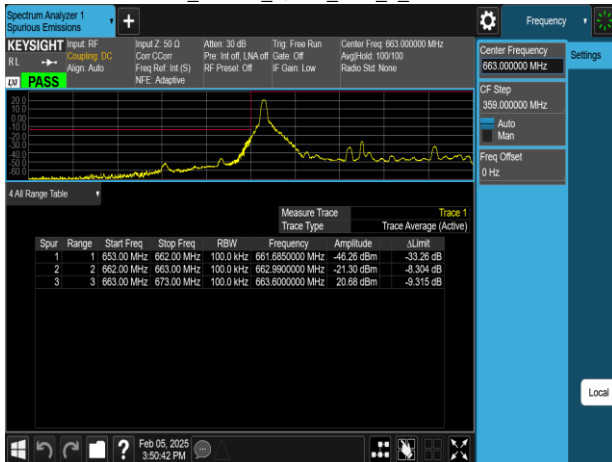
Band71_10MHz_QPSK_RB1_0_CH133172
