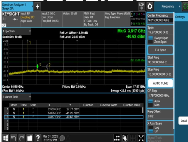
Band7_5MHz_QPSK_RB1_0_CH21100_below 18G
