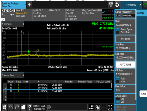
Band7_5MHz_QPSK_RB1_0_CH20775_upper 18G
