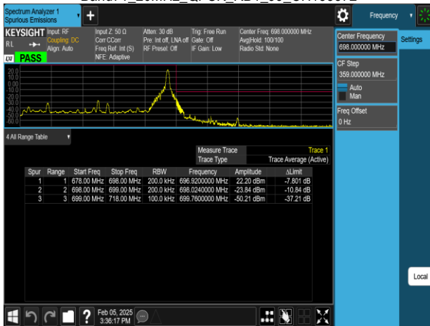
Band71_20MHz_QPSK_RB100_0_CH133372
