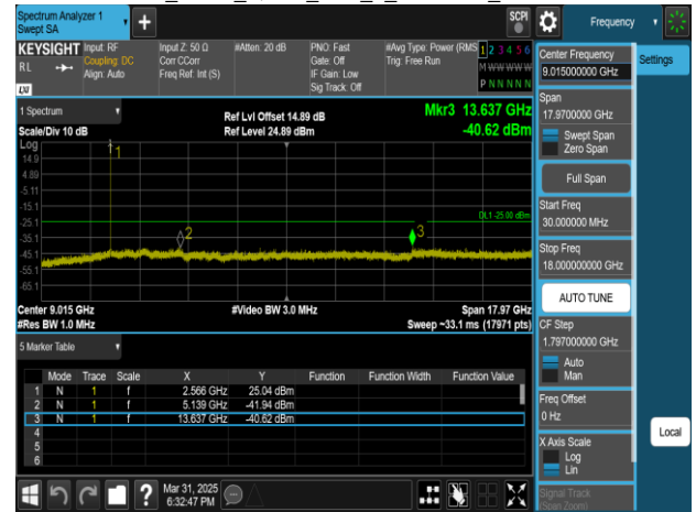
Band7_5MHz_QPSK_RB1_0_CH21425_upper 18G
