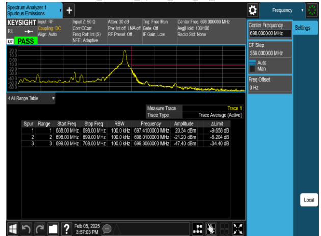
Band71_10MHz_QPSK_RB50_0_CH133422
