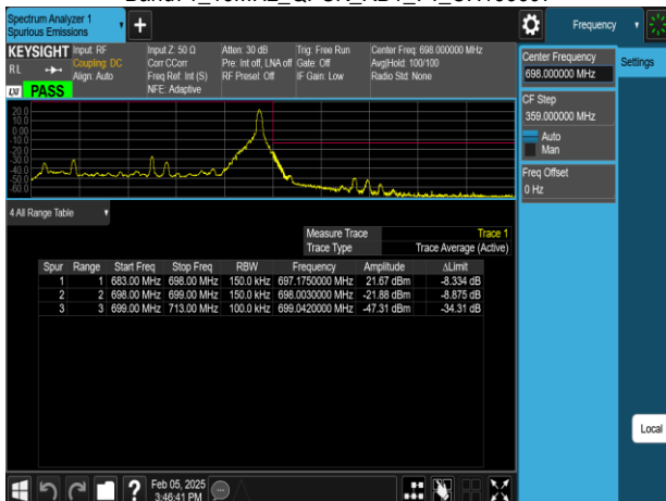
Band71_15MHz_QPSK_RB1_74_CH133397
