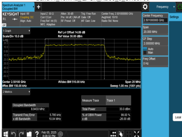
Band41_10MHz_QPSK_RB50_0_CH39700
