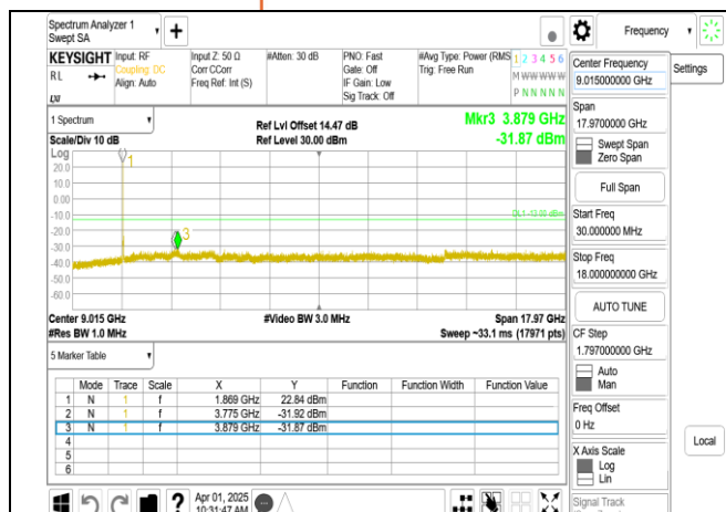
Band2_20MHz+20MHz_QPSK_RB1-99_1-0_CH18700-18898_low 18G
