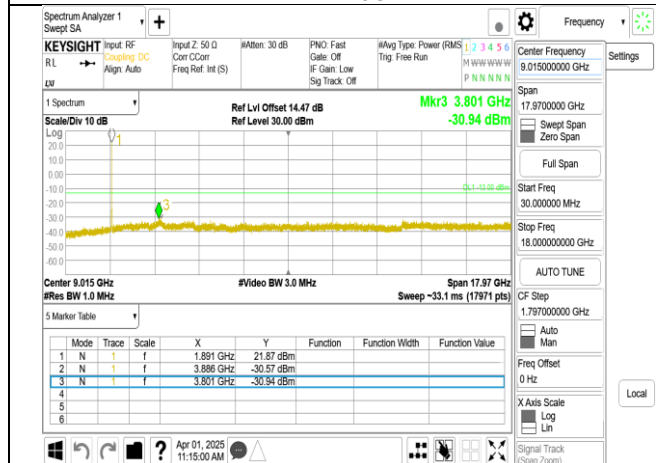
Band2_20MHz+20MHz_QPSK_RB1-99_1-0_CH18902-19100_low 18G
