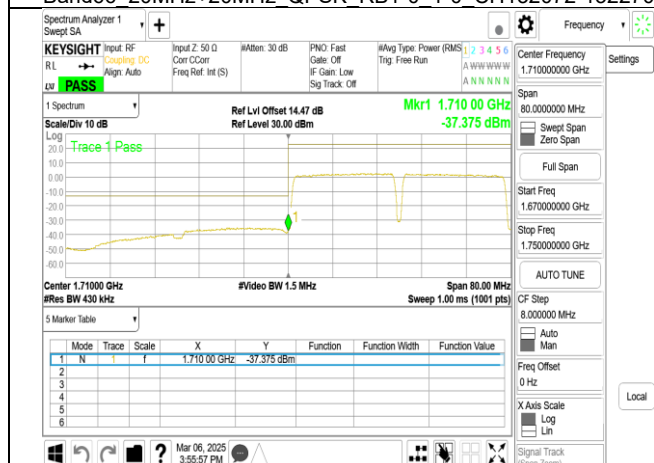
Band66_20MHz+20MHz_QPSK_RB100-0_100-0_CH132072-132270
