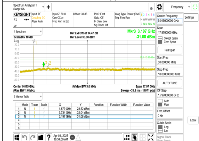
Band2_20MHz+20MHz_QPSK_RB1-99_1-0_CH18801-18999_low 18G
