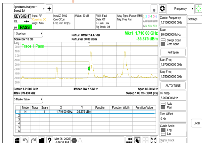
Band66_20MHz+20MHz_QPSK_RB1-0_1-0_CH132072-132270
