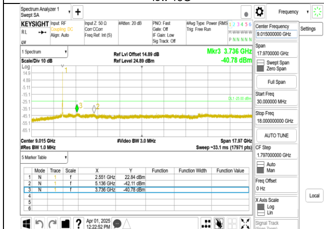
Band7_20MHz+20MHz_QPSK_RB1-99_1-0_CH21152-21350_low 18G
