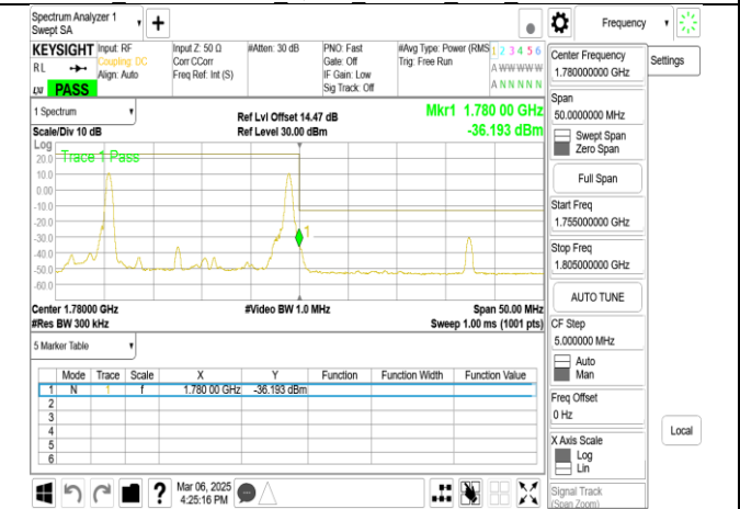
Band66 5MHz+20MHz QPSK RB1-25 1-99 CH132455-132572
