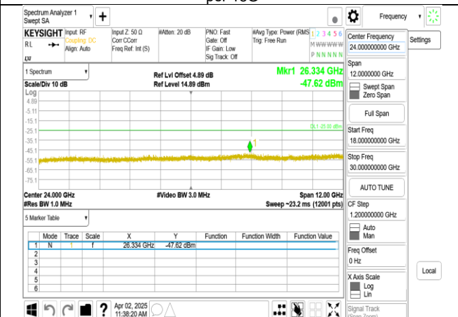
Band7_20MHz+20MHz_QPSK_RB1-99_1-0_CH21152-21350_up per 18G
