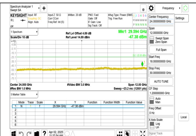
Band7_20MHz+20MHz_QPSK_RB1-99_1-0_CH20850-21048_up per 18G
