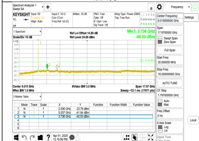
Band7_20MHz+20MHz_QPSK_RB1-99_1-0_CH21001-21199_low 18G
