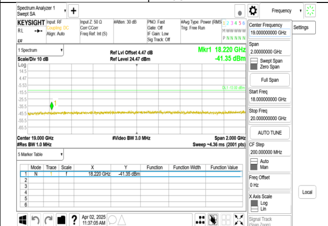
Band2_20MHz+20MHz_QPSK_RB1-99_1-0_CH18902-19100_up per 18G
