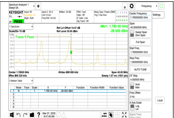
Band66B 10MHz+10MHz QPSK RB1-49 1-49 CH132523-132622
