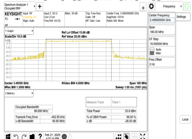
Band77-Part27_90MHz_DFT_s_OFDM_SCS30kHz_QPSK_RB243_0_CH633000
