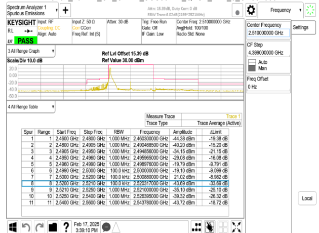
Band7_20MHz_CP_OFDM_SCS30kHz_QPSK_RB1_50_CH502000
