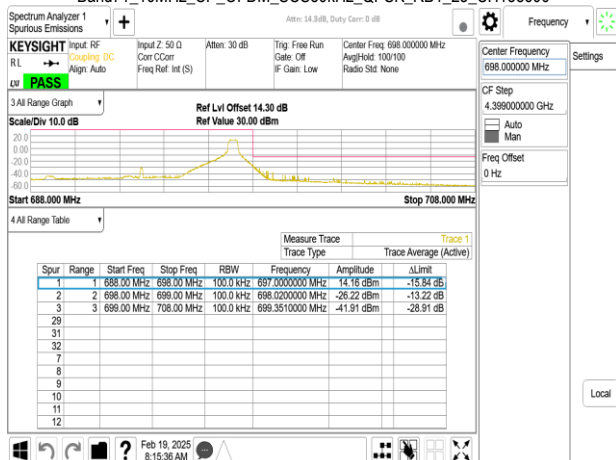
Band71_10MHz_CP_OFDM_SCS30kHz_QPSK_RB24_0_CH138600
