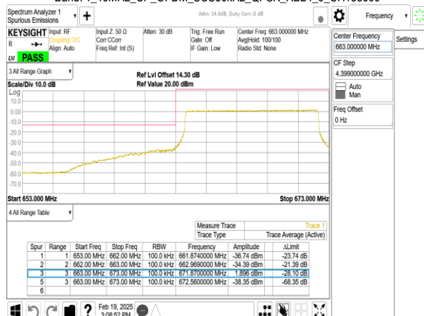
Band71_10MHz_CP_OFDM_SCS30kHz_QPSK_RB24_0_CH133600
