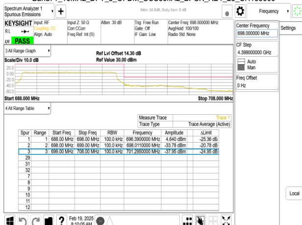
Band71_10MHz_DFT_s_OFDM_SCS30kHz_BPSK_RB1_23_CH138600
