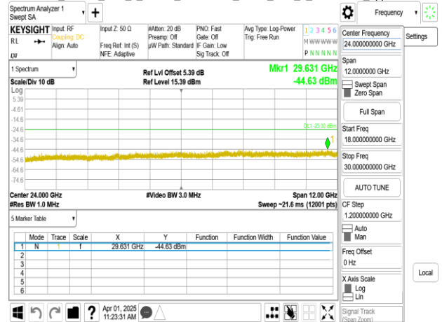
Band7_25MHz_DFT_s_OFDM_SCS30kHz_BPSK_RB1_1_CH507000_upper 18G
