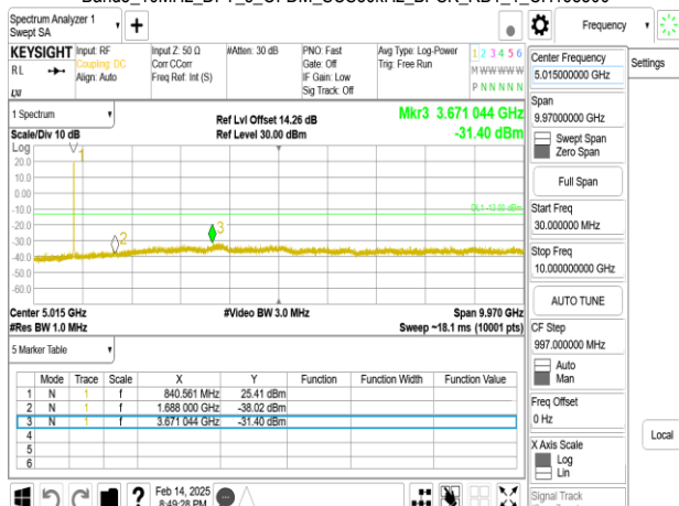
Band5_10MHz_DFT_s_OFDM_SCS30kHz_BPSK_RB1_1_CH168800
