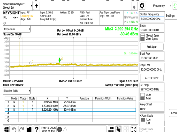
Band5_15MHz_DFT_s_OFDM_SCS15kHz_BPSK_RB1_1_CH168300
