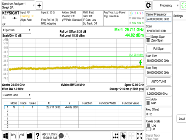
Band7_5MHz_DFT_s_OFDM_SCS15kHz_BPSK_RB1_1_CH507000_upper 18G
