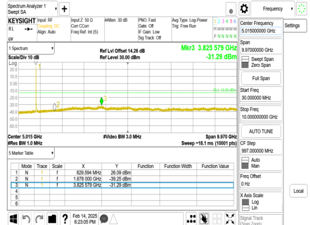
Band5_20MHz_DFT_s_OFDM_SCS15kHz_BPSK_RB1_1_CH168300
