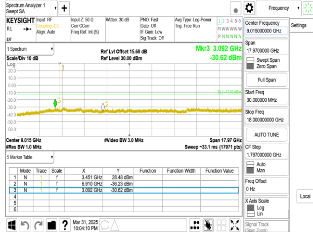
Band77-Part27_10MHz_DFT_s_OFDM_SCS30kHz_BPSK_RB1_1_CH633334_below 18G
