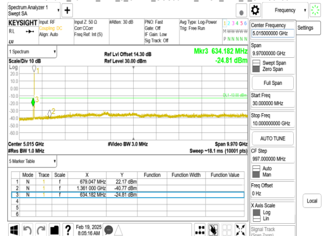
Band71_10MHz_DFT_s_OFDM_SCS30kHz_BPSK_RB1_1.CH136600
