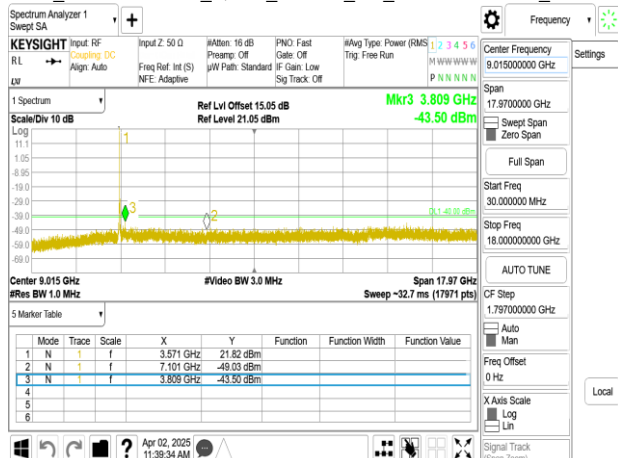
Band48_20MHz+20MHz_QPSK_RB1-99_1-0_CH55340-55538_upper 18G
