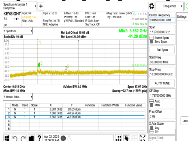
Band48_20MHz+20MHz_QPSK_RB1-99_1-0_CH56442-56640_upper 18G
