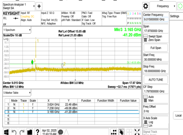
Band48_20MHz+20MHz_QPSK_RB1-99_1-0_CH55891-56089_below 18G
