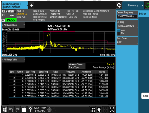
Band48_15MHz_QPSK_RB1_74_CH55315
