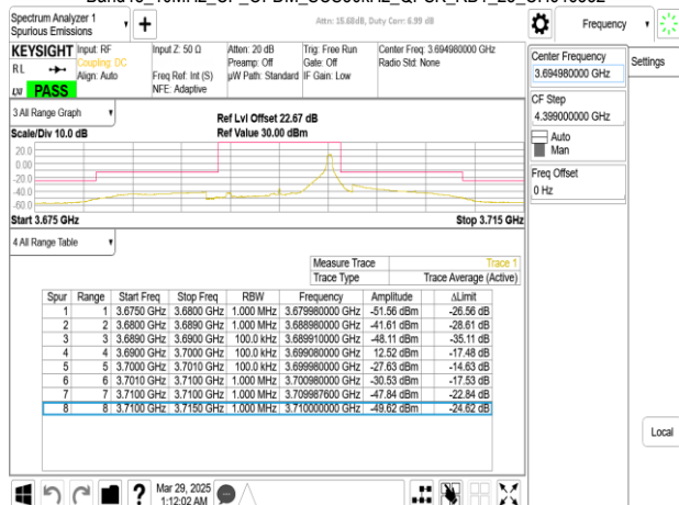
Band48_10MHz_CP_OFDM_SCS30kHz_QPSK_RB24_0_CH646332
