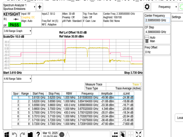
Band48_20MHz+20MHz_QPSK_RB100-0_100-0_CH56442-56640
