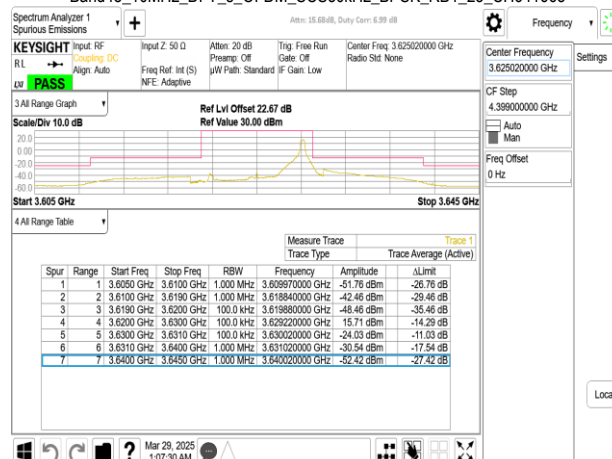
Band48_10MHz_DFT_s_OFDM_SCS30kHz_BPSK_RB1_23_CH641668
