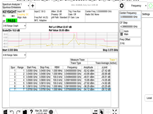
Band48_10MHz_DFT_s_OFDM_SCS30kHz_BPSK_RB1_23_CH637000
