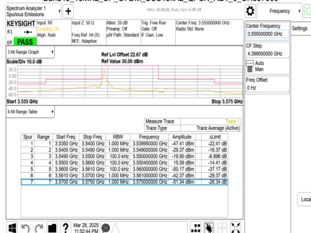
Band48_10MHz_CP_OFDM_SCS15kHz_QPSK_RB52_0_CH637000
