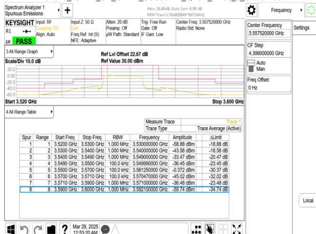
Band48_15MHz_CP_OFDM_SCS30kHz_QPSK_RB1_37_CH646166
