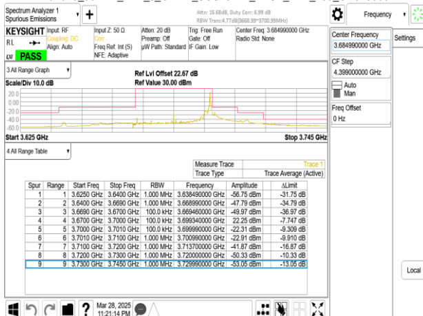
Band48_30MHz_DFT_s_OFDM_SCS15kHz_BPSK_RB1_159_CH645666
