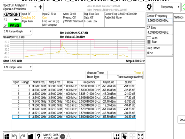
Band48_20MHz_DFT_s_OFDM_SCS30kHz_BPSK_RB1_0_CH673334
