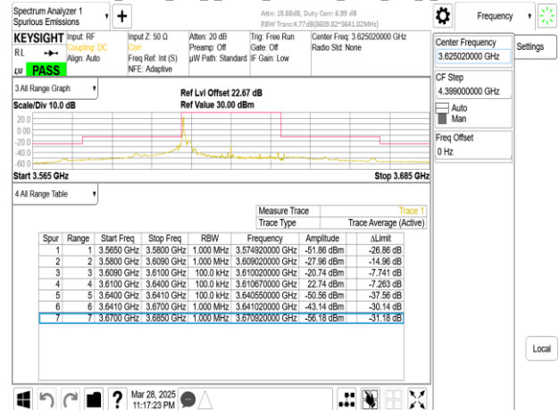
Band48_30MHz_DFT_s_OFDM_SCS15kHz_BPSK_RB1_159_CH641668
