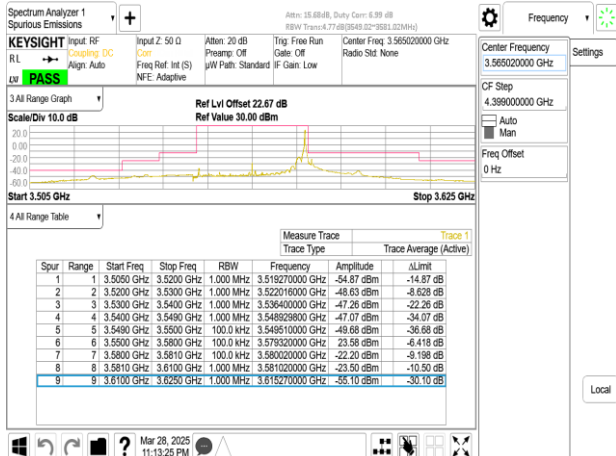
Band48_30MHz_DFT_s_OFDM_SCS15kHz_BPSK_RB1_159_CH637668
