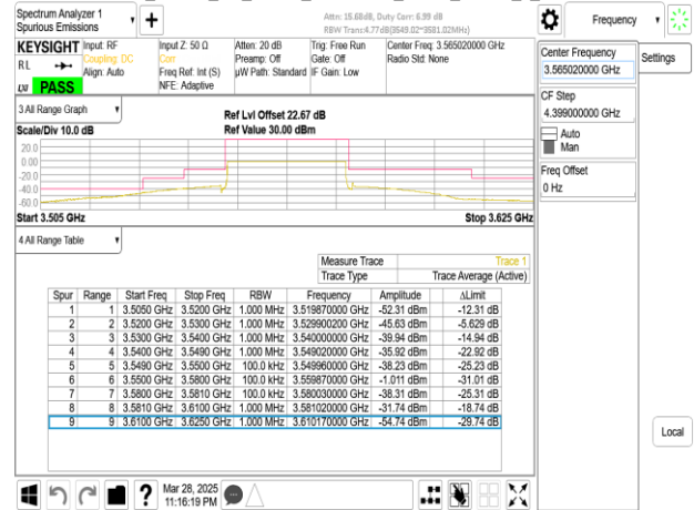
Band48_30MHz_CP_OFDM_SCS15kHz_QPSK_RB1_0_CH637668
