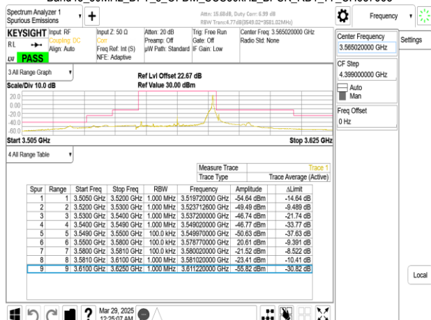
Band48_30MHz_DFT_s_OFDM_SCS30kHz_BPSK_RB1_77_CH637668
