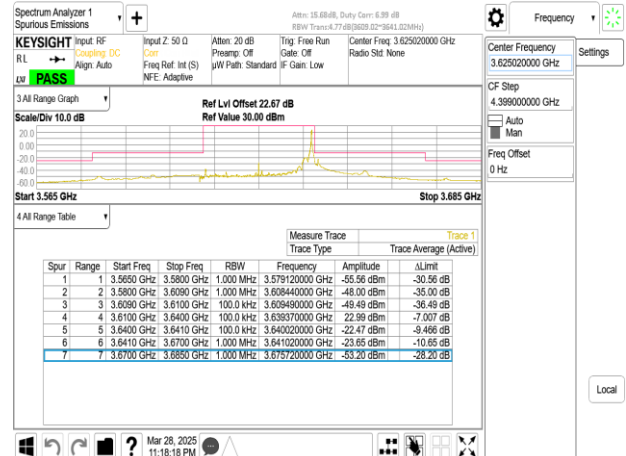
Band48_30MHz_DFT_s_OFDM_SCS15kHz_BPSK_RB1_159_CH641668
