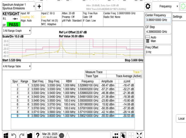
Band48_20MHz_CP_OFDM_SCS30kHz_QPSK_RB1_0_CH637334
