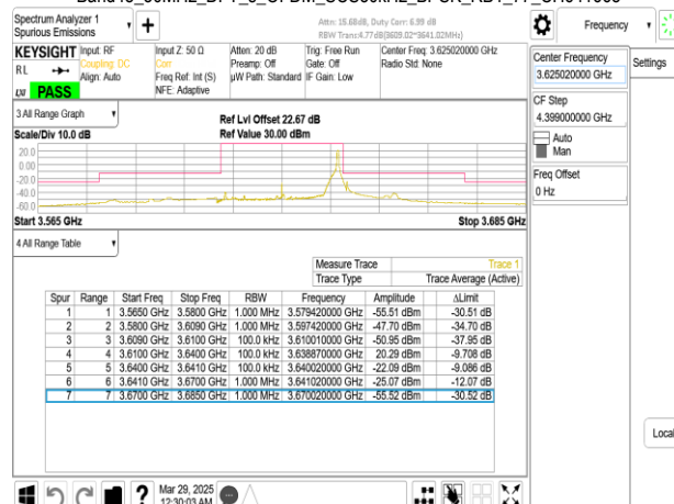
Band48_30MHz_DFT_s_OFDM_SCS30kHz_BPSK_RB1_77_CH641668
