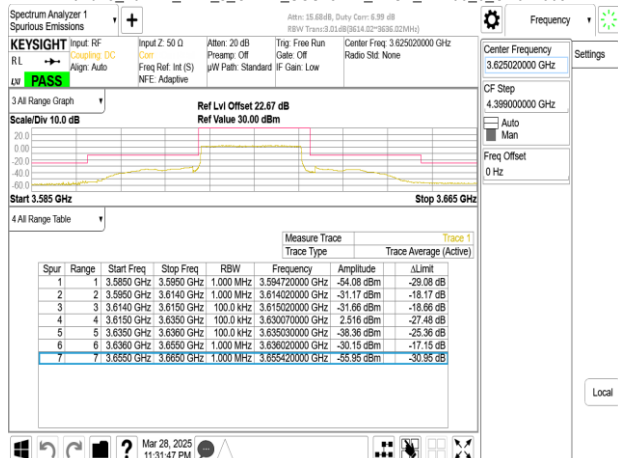
Band48_20MHz_DFT_s_OFDM_SCS15kHz_BPSK_RB1_0_CH641668
