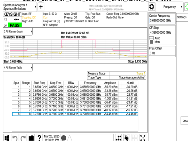
Band48_20MHz_CP_OFDM_SCS15kHz_QPSK_RB1_105_CH646000
