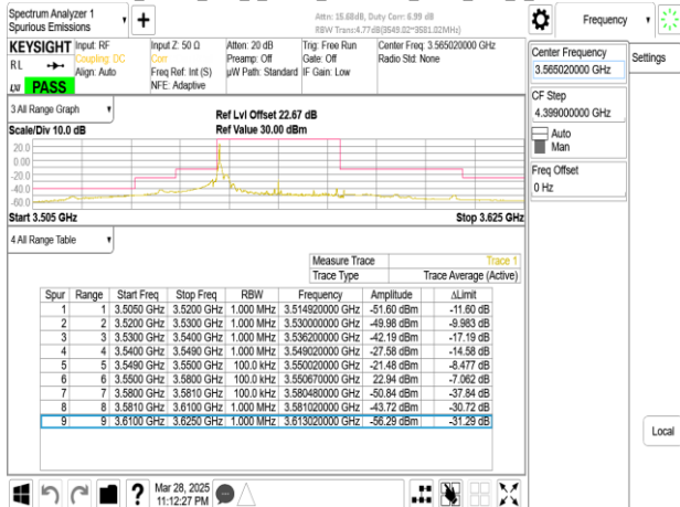
Band48_30MHz_DFT_s_OFDM_SCS15kHz_BPSK_RB1_159_CH637668
