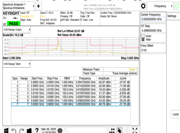
Band48_20MHz_DFT_s_OFDM_SCS15kHz_BPSK_RB1_0_CH641668
