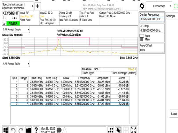
Band48_20MHz_DFT_s_OFDM_SCS30kHz_BPSK_RB1_0_CH641668
