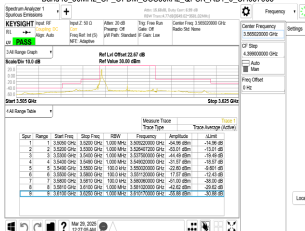
Band48_30MHz_CP_OFDM_SCS30kHz_QPSK_RB78_0_CH637668
