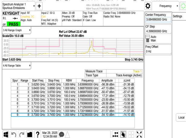
Band48_30MHz_CP_OFDM_SCS30kHz_QPSK_RB78_0_CH645666
