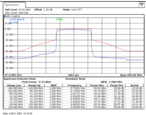
802.11ax80 / 6865MHz / Chain D - CDD
