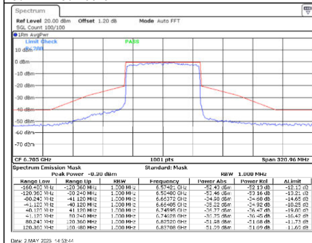
802.11ax80 / 6705MHz / Chain A - CDD
