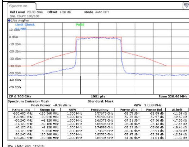
802.11ax80 / 6705MHz / Chain C - CDD
