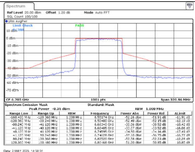
802.11ax80 / 6705MHz / Chain D - CDD
