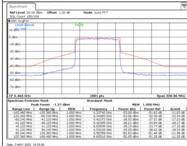
802.11ax80 / 6465MHz / Chain A - CDD
