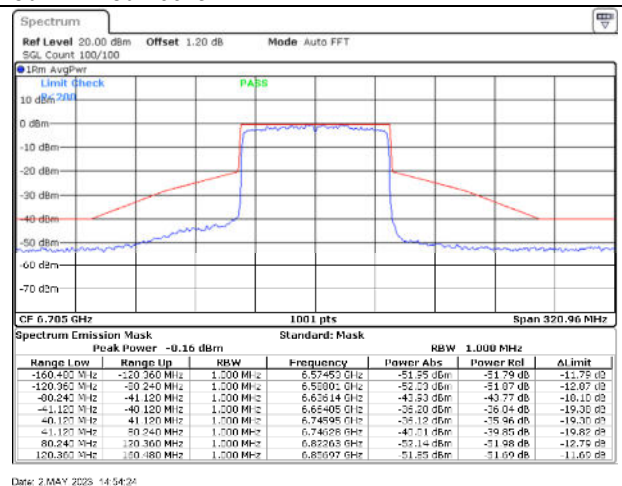
802.11ax80 / 6705MHz / Chain B - CDD
