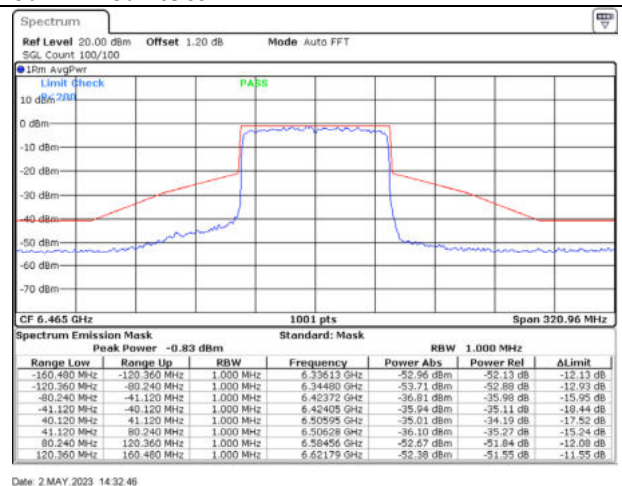
802.11ax80 / 6465MHz / Chain B - CDD
