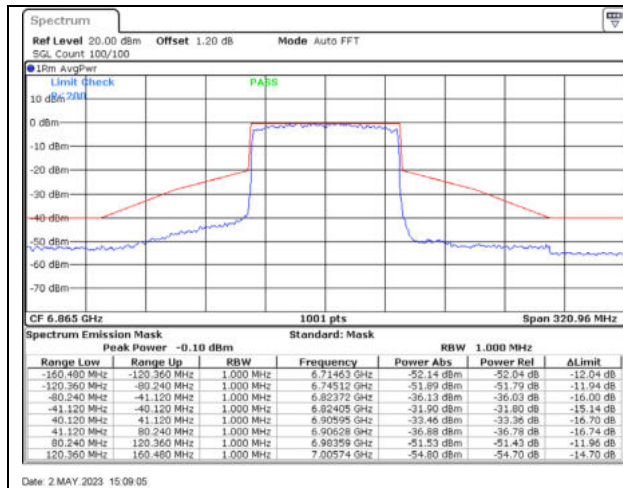
802.11ax80 / 6865MHz / Chain C - CDD
