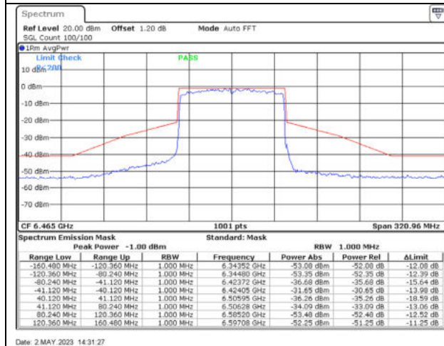
802.11ax80 / 6465MHz / Chain C - CDD
