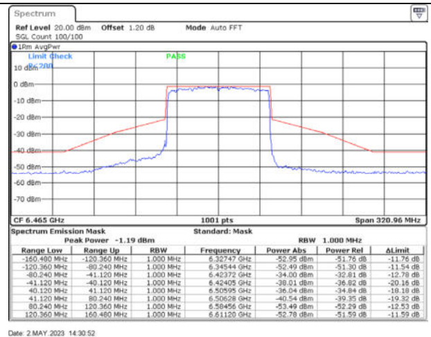
802.11ax80 / 6465MHz / Chain D - CDD
