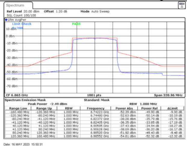
802.11ax80 / 6865MHz / Chain D - Beamforming
