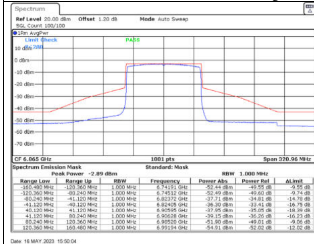
802.11ax80 / 6865MHz / Chain C - Beamforming
