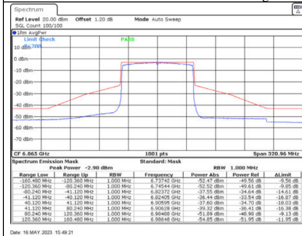
802.11ax80 / 6865MHz / Chain A - Beamforming
