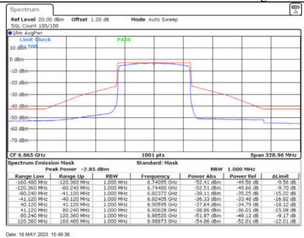
802.11ax80 / 6865MHz / Chain B - Beamforming
