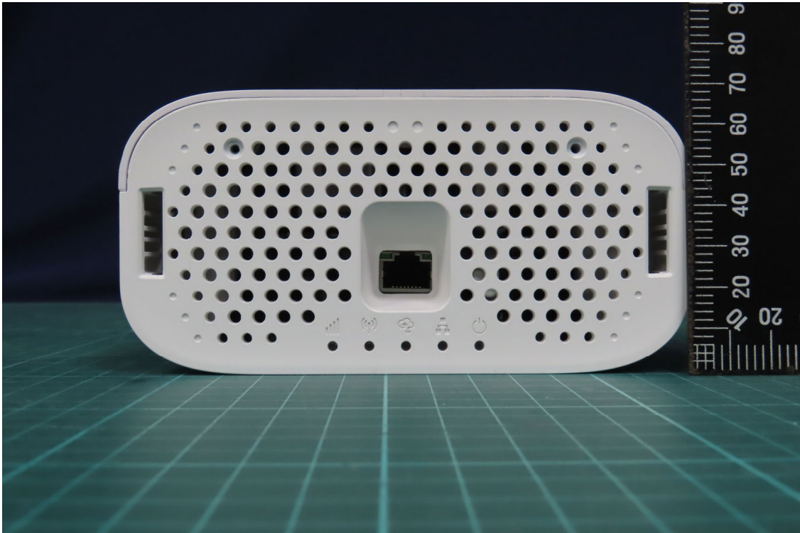
(5) EUT Photo
