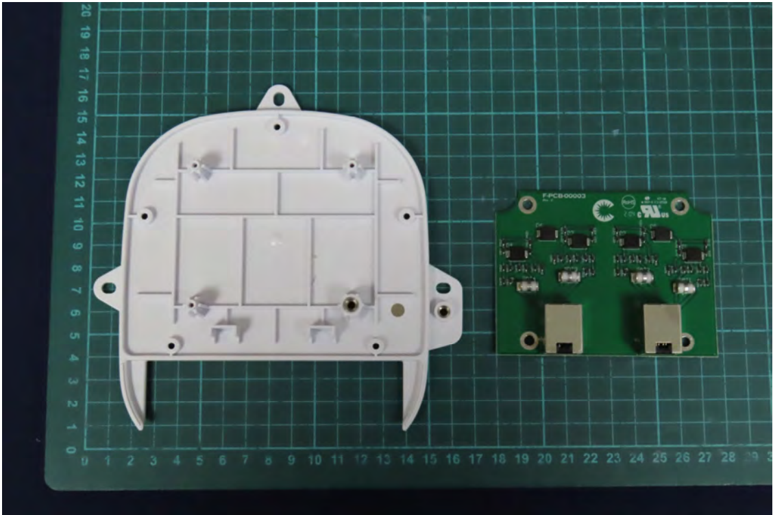
(74) EUT Photo
