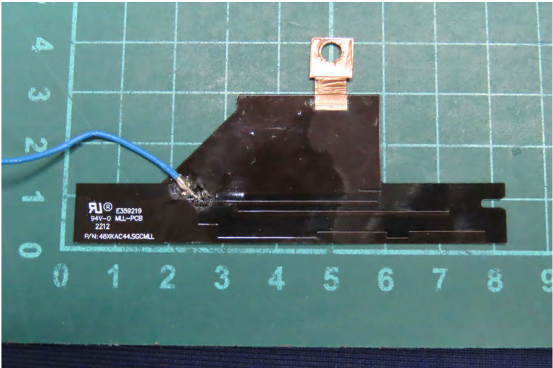
(59) EUT Photo_ LTE/FR1 Ant 3
