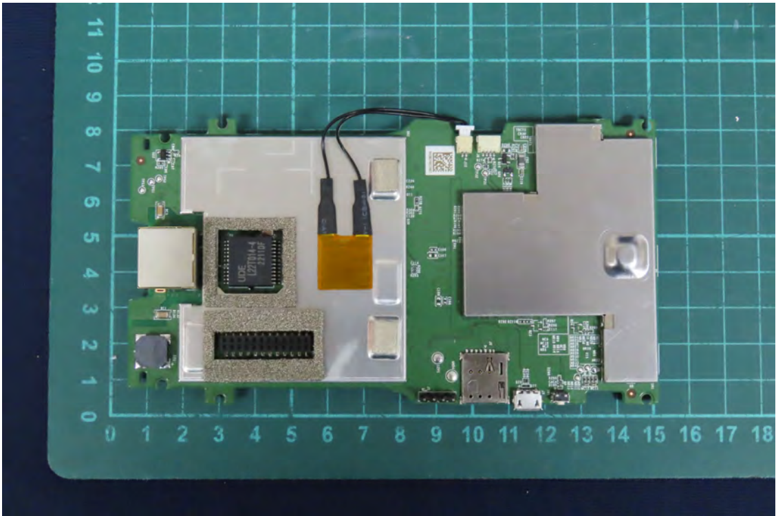
(33) EUT Photo
