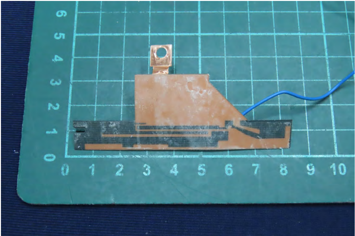
(60) EUT Photo_ LTE/FR1 Ant 3
