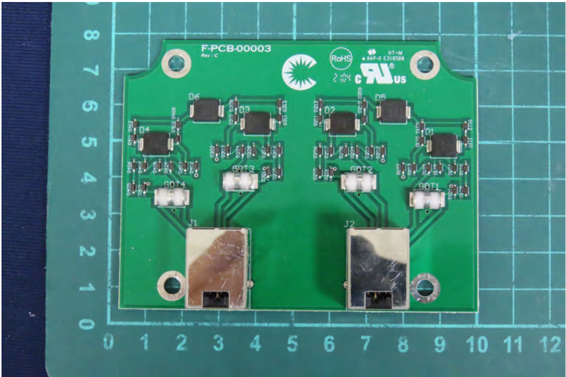
(75) EUT Photo
