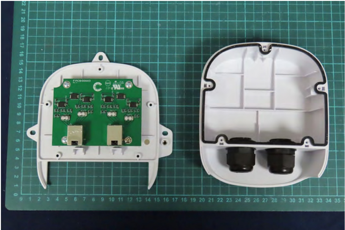
(72) EUT Photo
