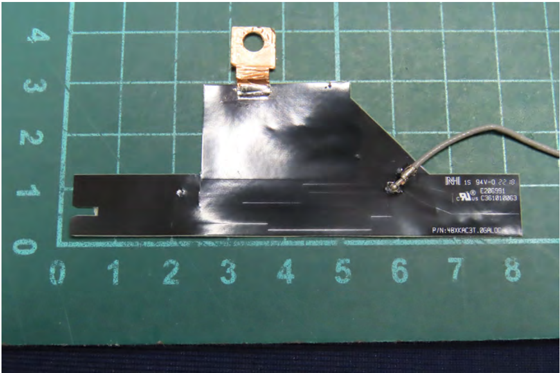
(61) EUT Photo_ LTE/FR1 Ant 1
