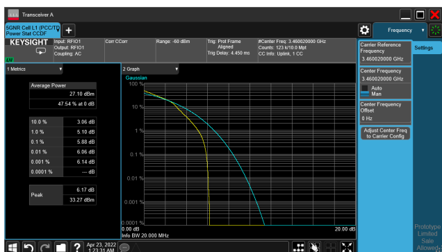
5G NR n77_CH633334_20M_1RB_QPSK_Ratio
