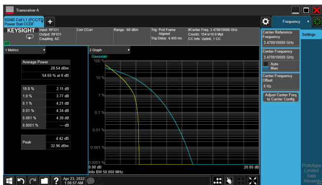
5G NR n77_CH631334_40M_1RB_16-QAM_Ratio
