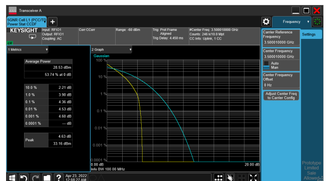
5G NR n77_CH633334_90M_1RB_16-QAM_Ratio
