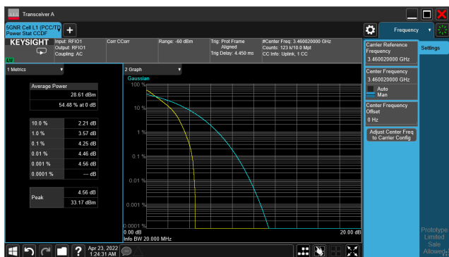
5G NR n77_CH630668_20M_1RB_16-QAM_Ratio
