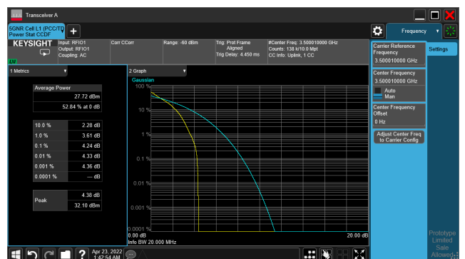
5G NR n77_CH633334_15M_1RB_16-QAM_Ratio
