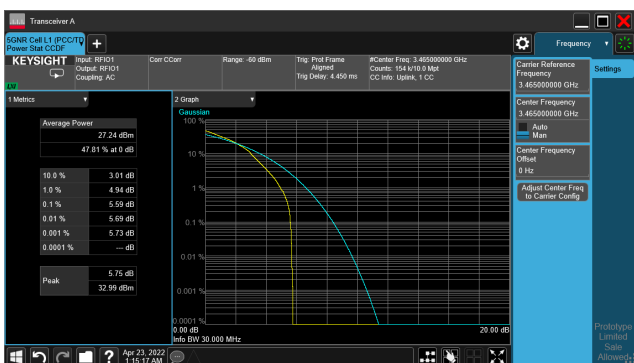
5G NR n77_CH633334_30M_1RB_QPSK_Ratio
