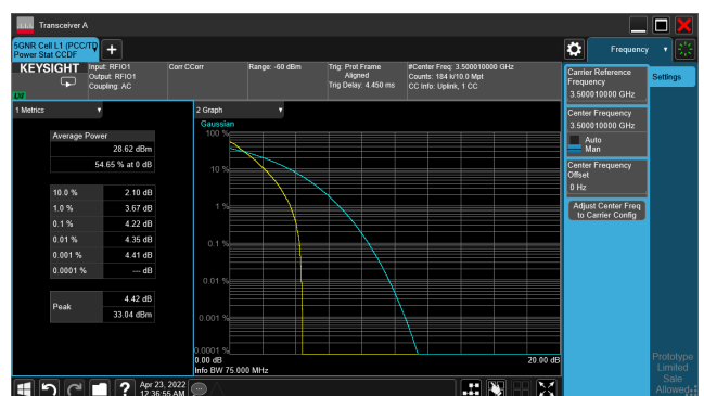
5G NR n77_CH633334_60M_1RB_16-QAM_Ratio
