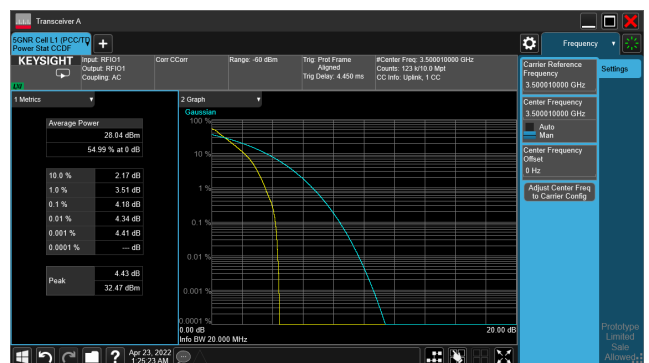
5G NR n77_CH633334_20M_1RB_16-QAM_Ratio
