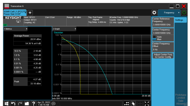
5G NR n77_CH633334_10M_1RB_16-QAM_Ratio
