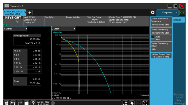
5G NR n77_CH633334_30M_1RB_16-QAM_Ratio
