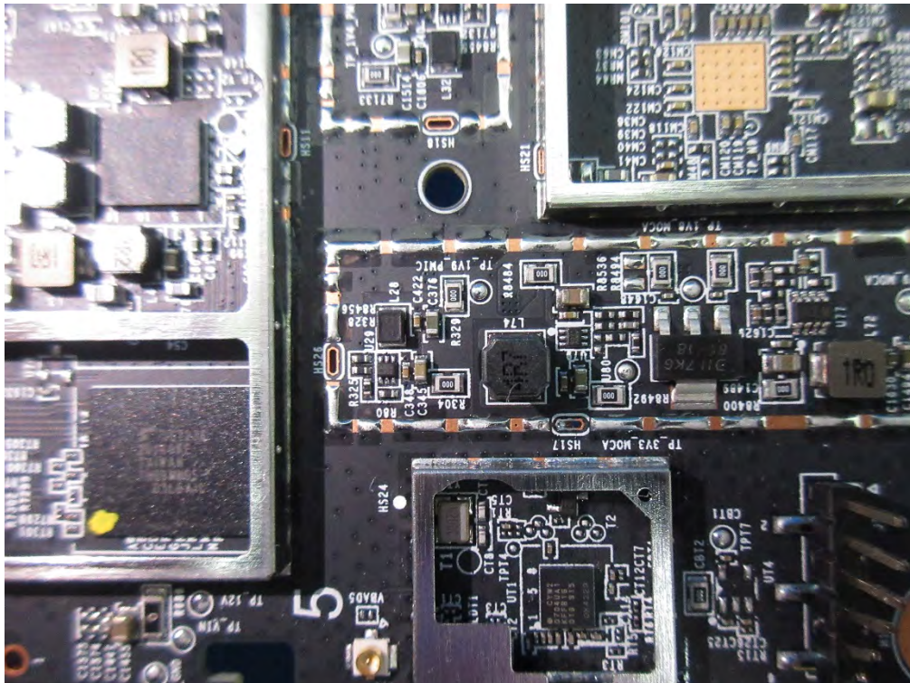
(109) EUT Photo
