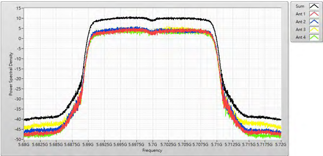
Channel 140 (5700MHz)
